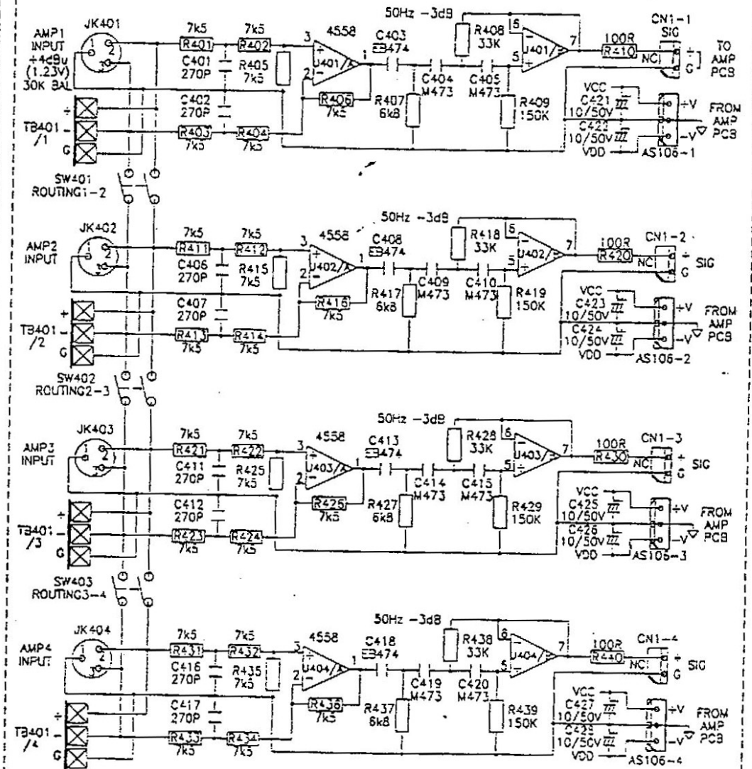
PCB SUB(3):JPA-4C-C (INPUT)
