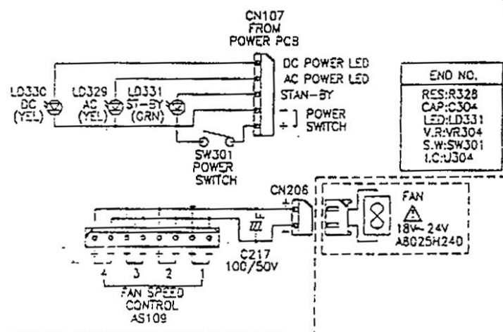
PCB SUB(4):JPA-4C-D (OUTPUT TERMINAL)
