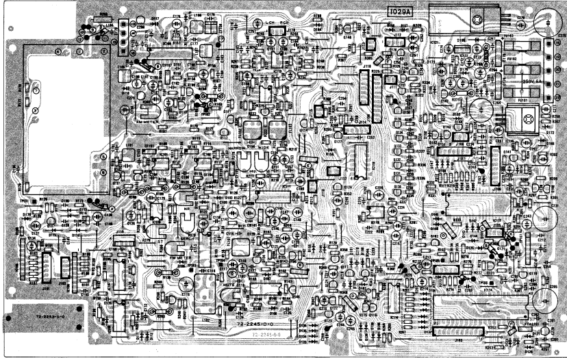
TUNER P.C.B. ASS'Y (I029A)
