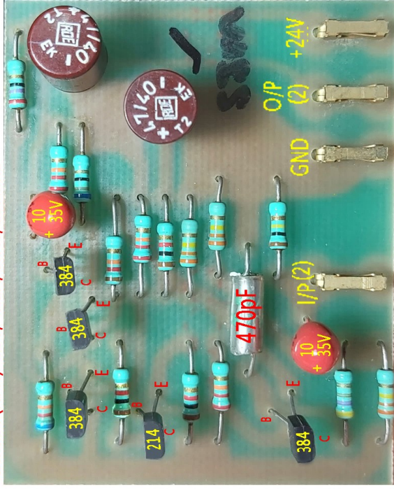
ZTX384 (NPN) 30V, 0.2A, 0.5W, 150MHz ZTX384 (NPN) -30V, -0.2A, 0.5W, 150MHz
