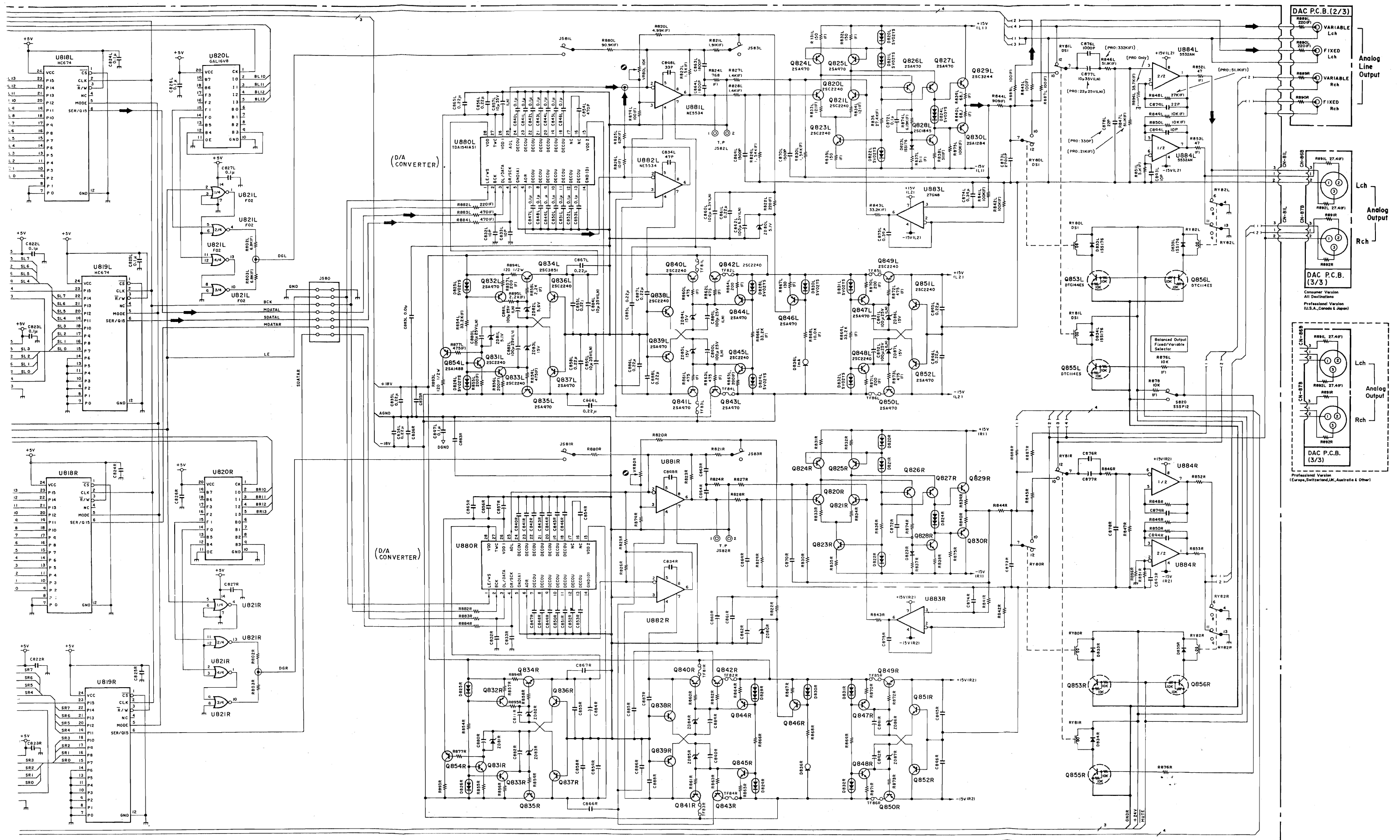
Fig. 9.2 DAC Section
