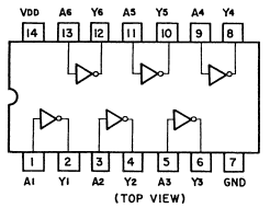
Fig. 13.8 Inverter C-MOS IC μPD4049C
