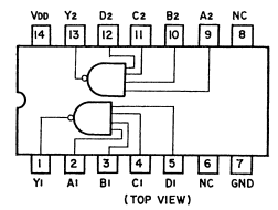
Fig. 13.16 NAND Gate C-MOS IC μPD4012C
