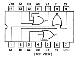
Fig. 13.13 NOR Gate C-MOS IC μPD4025C
