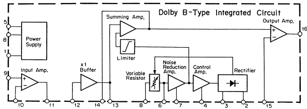
Fig. 13.4 Dolby NR IC μA7300PC
