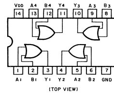
Fig. 13.11 OR Gate C-MOS IC μPD4071C
