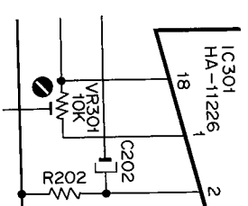
Fig. 4.10 Dolby NR Circuit
