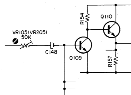
Fig. 7.1 2. Meter Level
