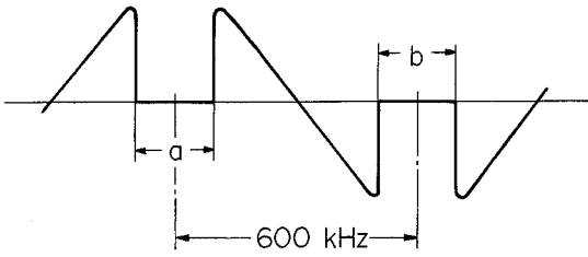
Fig. 4.1.4 S-Curve
