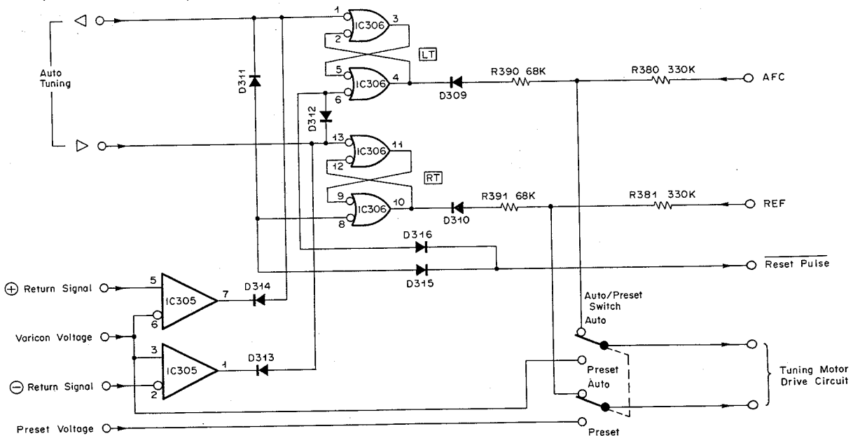
Fig. 2.3.11 Auto-Tuning Circuit
