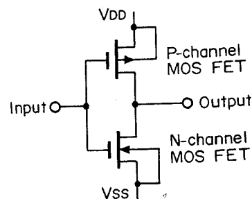
Fig. 2.1.1 C-MOS Inverter
