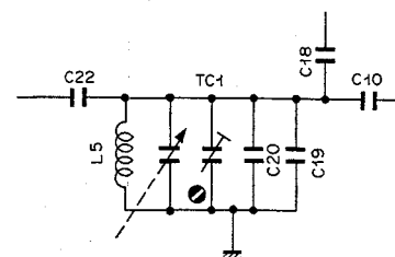
Fig. 4.1.11 12. Dial Calibration
