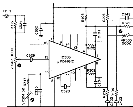
Fig. 4.1.9 8. Separation
