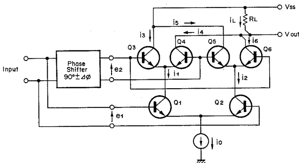
Fig. 2.1.17 Quadrature Detector Circuit
