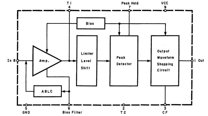
Fig. 8.1.10 Pre-amp. IC \mu PC1474HA
