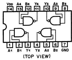
Fig. 8.1.3 NAND Gate C-MOS IC \mu PD4011BC
