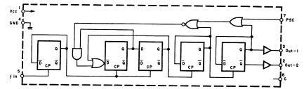
Fig. 7.1.12 ECL Prescaler (FM) IC TD6104P
