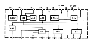
Fig. 7.1.11 AM Tuner IC LA1247
