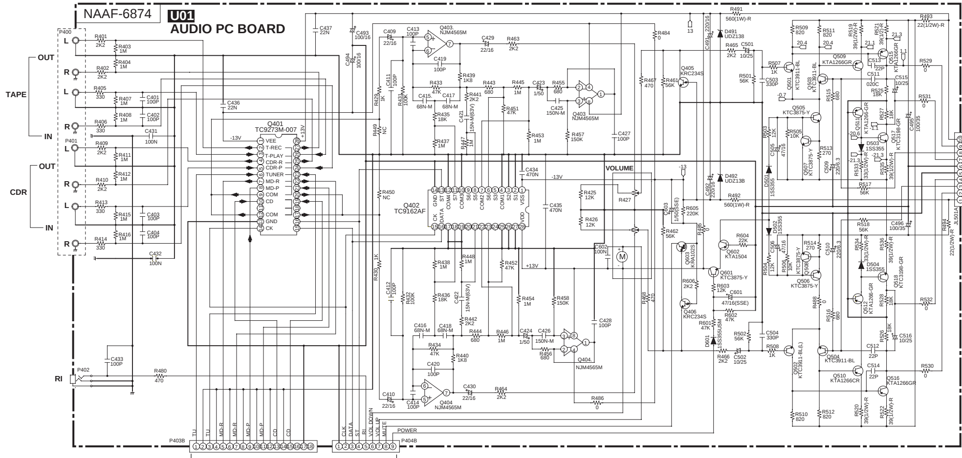
TO NAAR-6875 SCHEMATIC-DIAGRAMS-2
