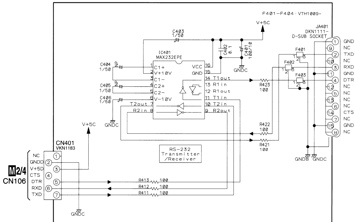
R 232B ASSY (VWG2129)
