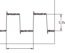
(WF07) DSP LRCK3
