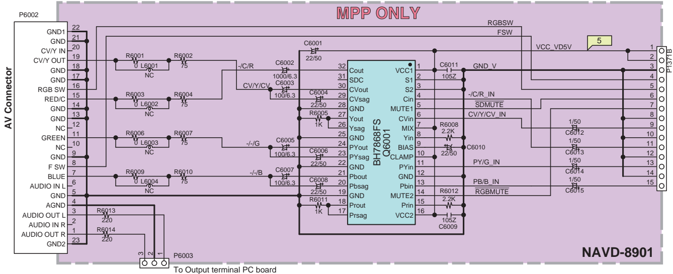
U07 : AV CONNECTOR PC BOARD
