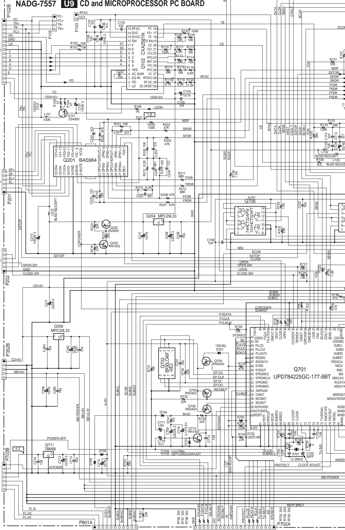
To NADIS-7586(P801) SCHEMATIC DIAGRAMS-3
