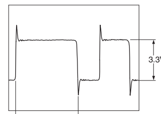
(WF03) SAI_SDOUT (SD-3 : E4)
