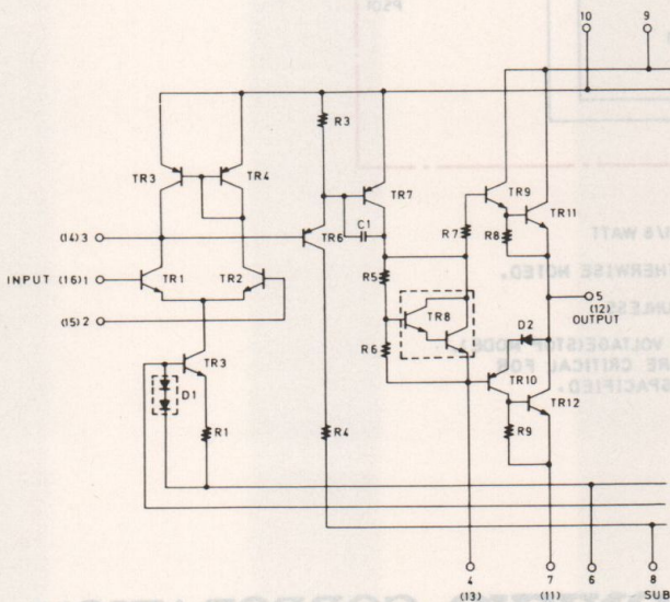
STK-4913 (Power amplifier)
