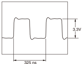
(WF08) BCK_GND_PLD (SD-12:I7)
