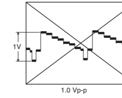
S-Video Y waveform (WF22)
