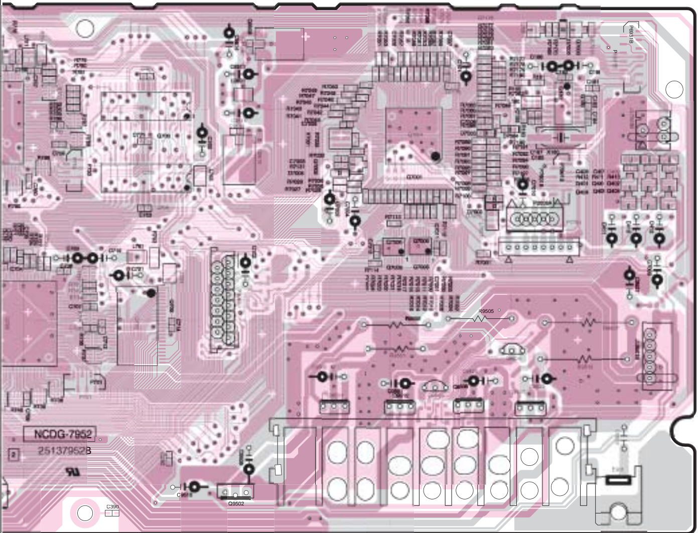
DSP CIRCUIT PC BOARD(NADG-7952)
