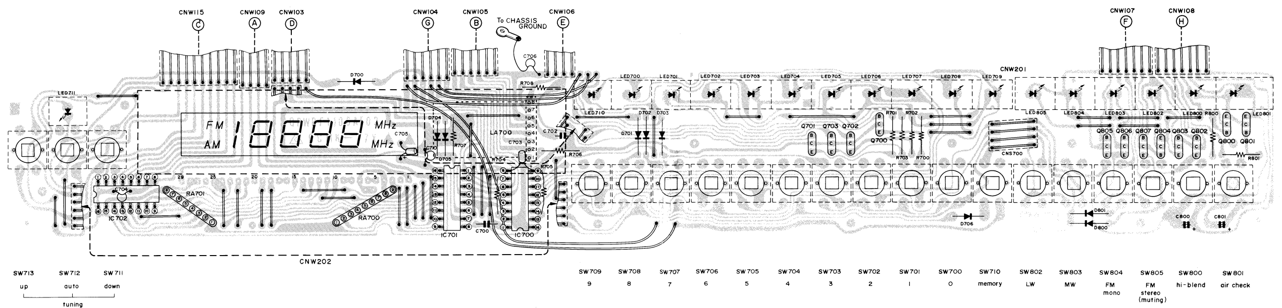
Abbildung 9 VERDRAHTUNGSSEITE DES FRONTBEDIENTUNGSKREISES (TASTATURMATRIX), DER ABSTIMMFREQUENZANZEIGE/FELDSTÄRKEANZEIGE UND DER SENDERFREQUENZ Figure 9 COTE CABLAGE DU CIRCUIT D'OPERATION AVANT (MATRICE A CLAVIER), AFFICHAGE DE FREQUENCE D'ACCORD/INDICATEUR DE PUISSANCE DU SIGNAL ET FREQUENCE DE STATION
