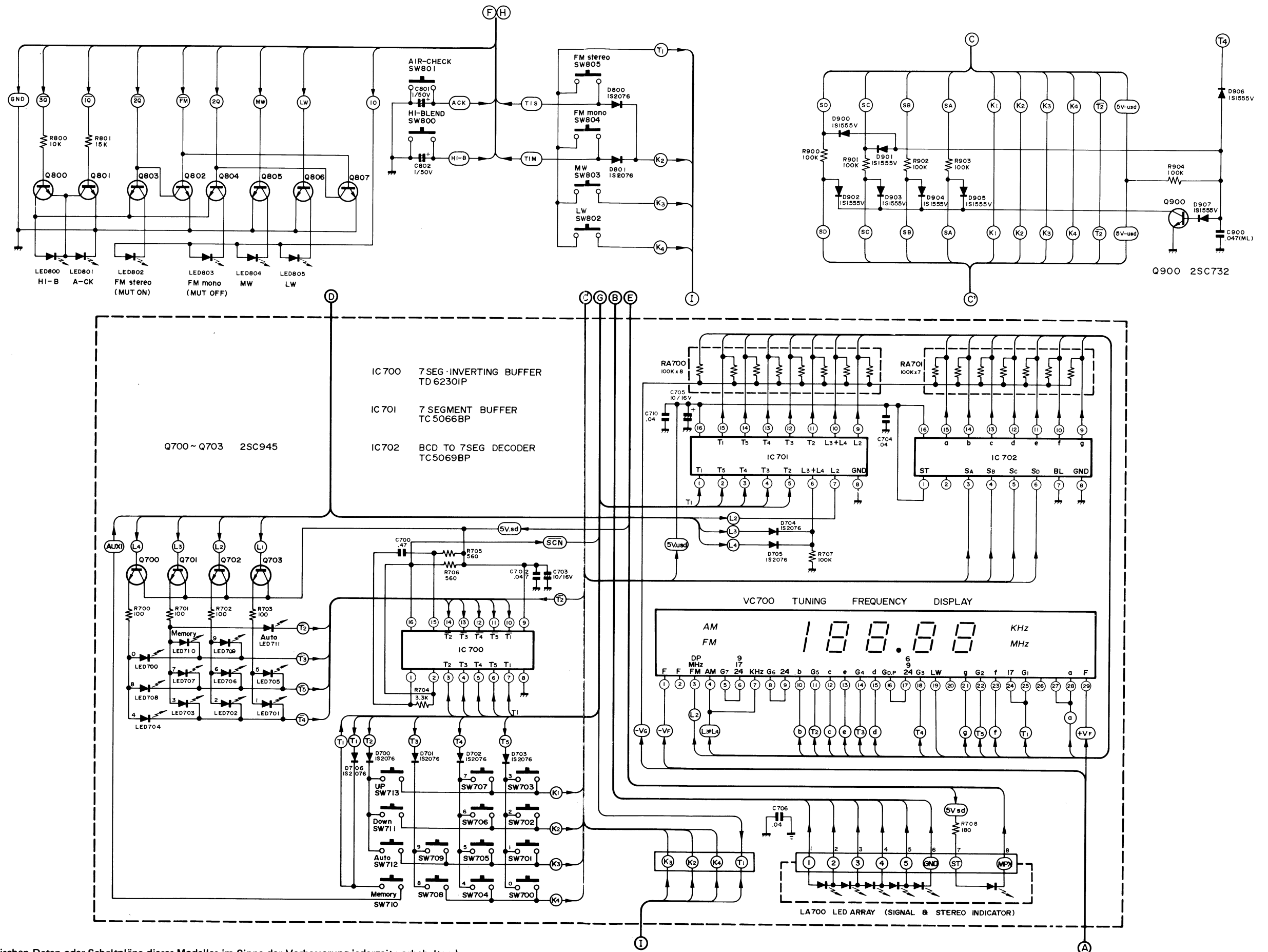
Abbildung 7 SCHEMATISCHER SCHALTPLAN DES FRONTBEDIENTUNGSKREISES (TASTATURMATRIX), DER SENDEFREQUENZANZEIGE/FELDESTÄRKEANZEIGE UND DER SENDEFREQUENZ Figure 7 DIAGRAMME SCHEMATIQUE DU CIRCUIT D'OPERATION AVANT (MATRICE A CLAVIER) INDICATEUR DE PUISSANCE DU SIGNAL ET FREQUENCE DE STATION
