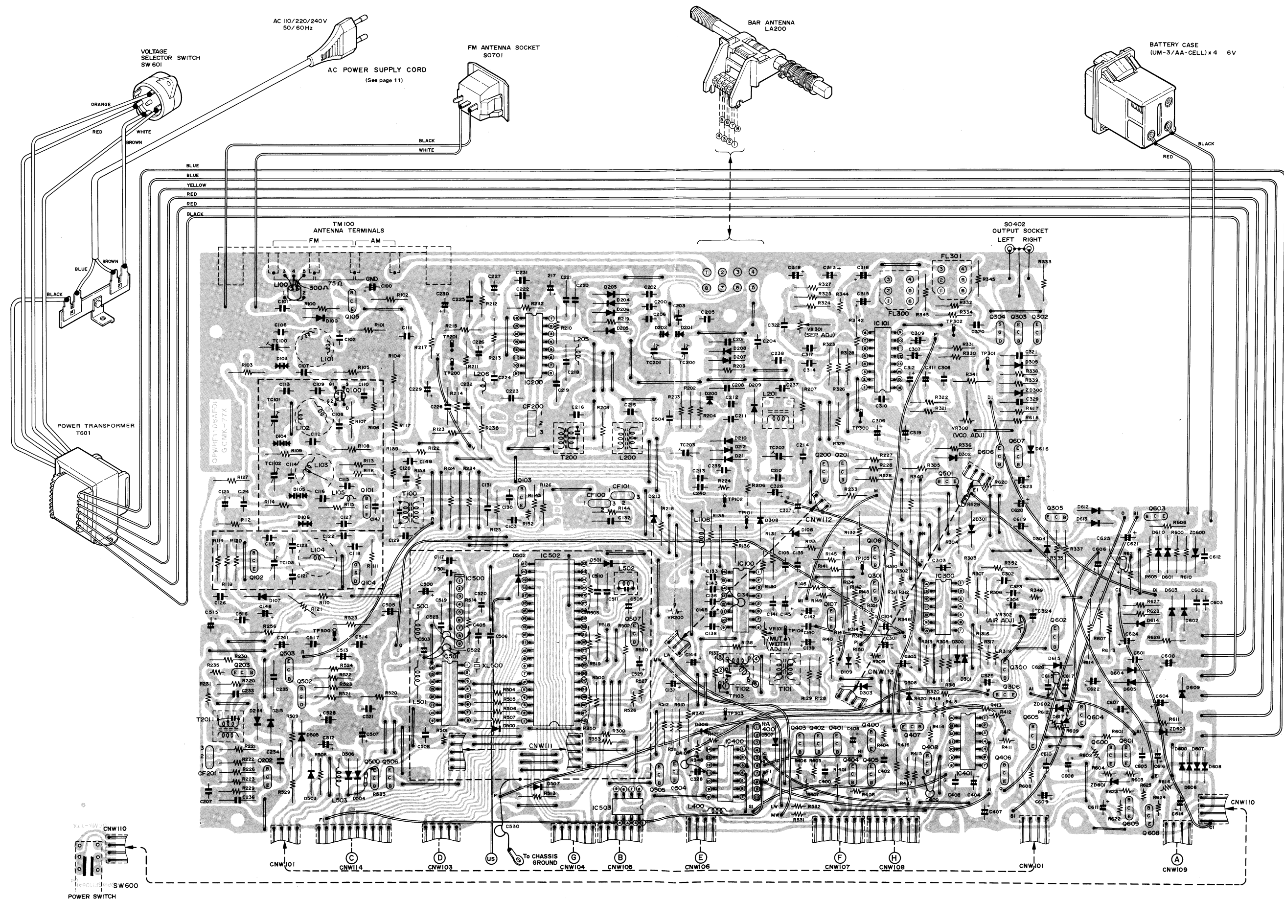
Abbildung 5 VERDRAHTUNGSSEITE DER LINEAR-/STROMVERSORUNGS-/HAUPTDIGITAL-/FREQUENZANZEIGEDIGITALKREISLEITERPLATTE Figure 5 COTE CABLE DE LA PMI DU CIRCUIT LINEAIRE/NUMERIQUE PRINCIPAL/NUMERIQUE D'AFFICHAGE DE FREQUENCE
