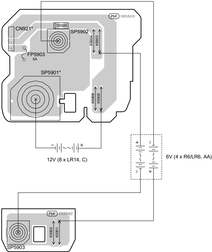
H BATTERY (1) P.C.B. (REPNT0063A...RX-D45EB/EG) (REPNT0063B...RX-D50EB/EG)
