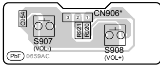
E VOLUME P.C.B. (REPNT0062A...RX-D45EB/EG) (REPNT0062B...RX-D50EB/EG)
