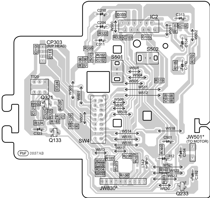
C DECK P.C.B. (REPNT0061AB...RX-D45EB/EG) (REPNT0061BB...RX-D50EG) (REPNT0061HB...RX-D50EB)
