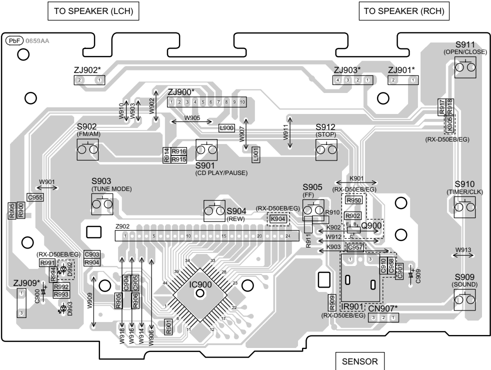
D PANEL P.C.B. (REPNT0062A...RX-D45EB/EG) (REPNT0062B...RX-D50EB/EG)
