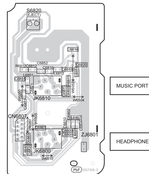
E MUSIC PORT P.C.B. (REPX0649E)
