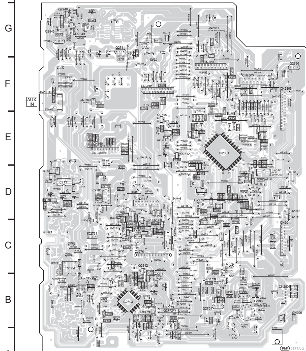
B MAIN P.C.B. (REPX0648E...PL) (REPX0648F...GCP)
