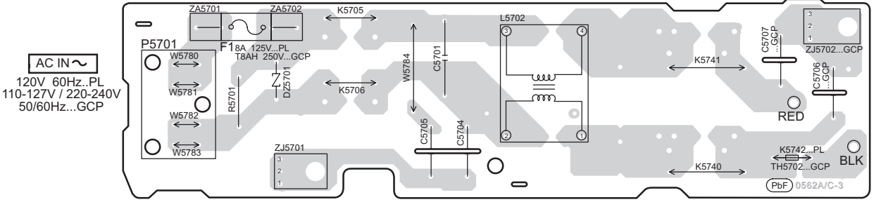
L AC INLET P.C.B. (REPX0676D...PL) (REPX0676E...GCP)
