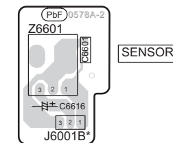
F REMOTE SENSOR P.C.B. (REPX0649E)
