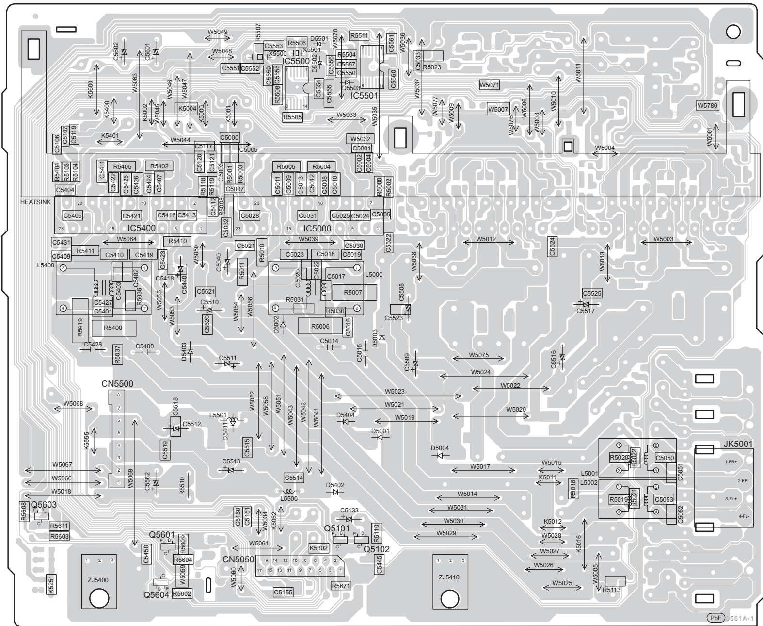
J D-AMP P.C.B (REPX0638A)
