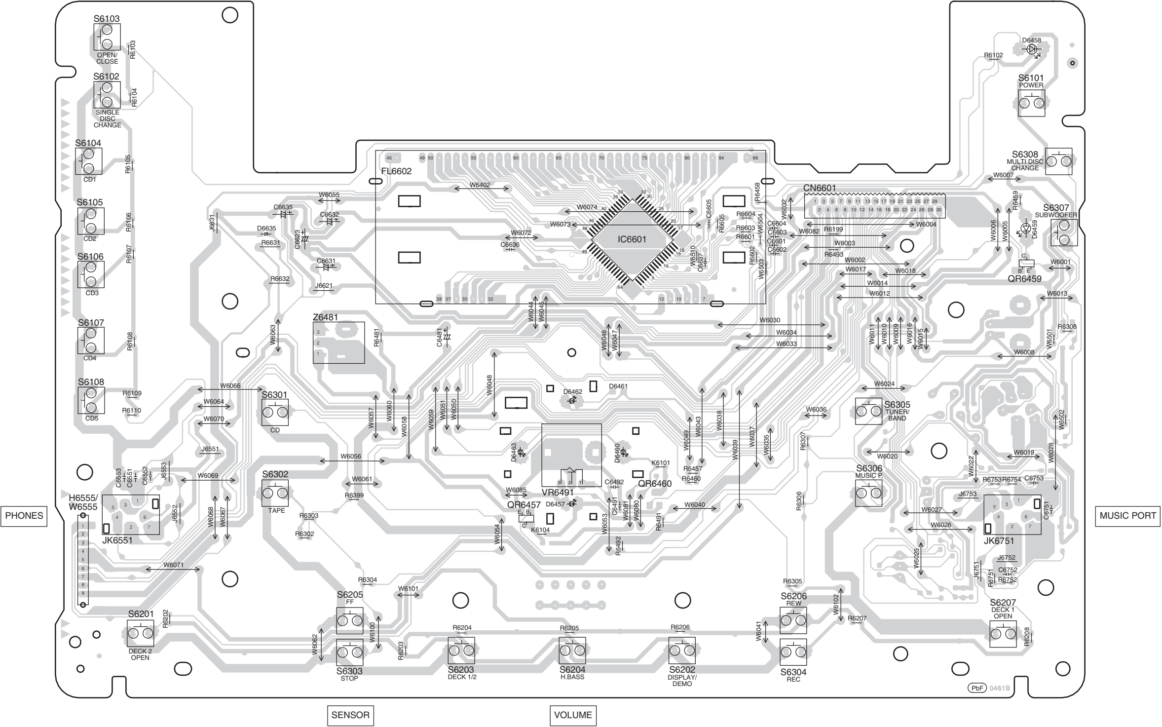
C PANEL P.C.B (REPX0517J)
