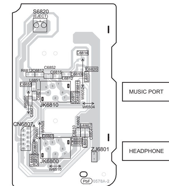
G MUSIC PORT P.C.B. (REPX0649C)
