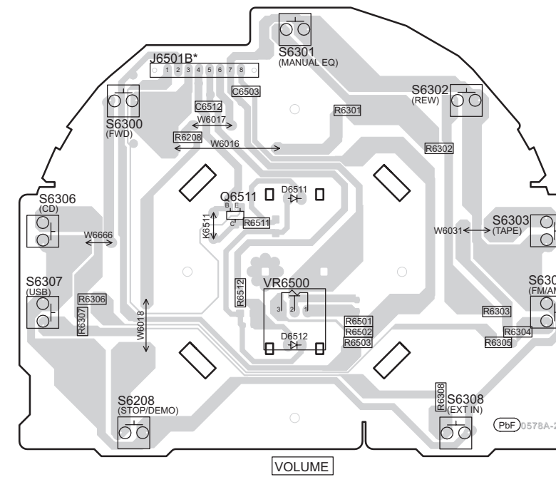
H REMOTE SENSOR P.C.B. (REPX0649C)
