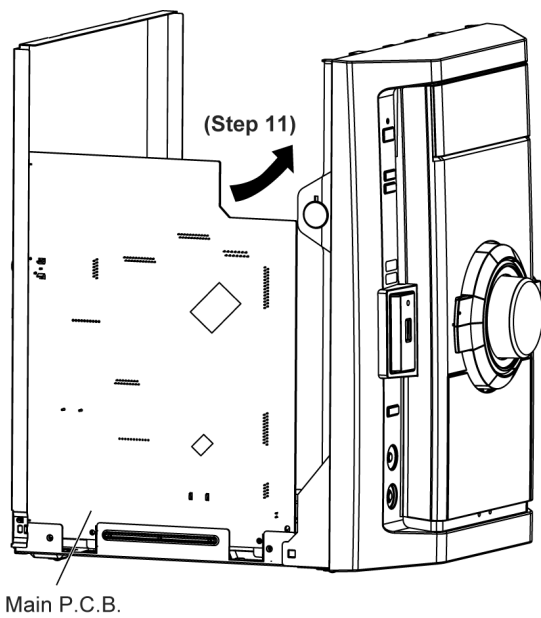
Main P.C.B.
