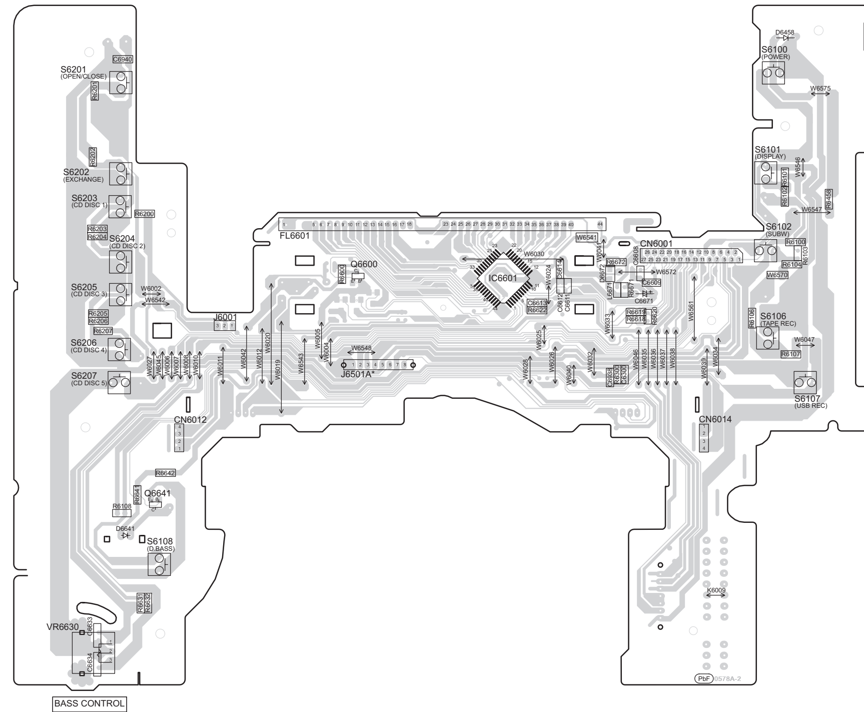
C PANEL P.C.B. (REPX0649C)
