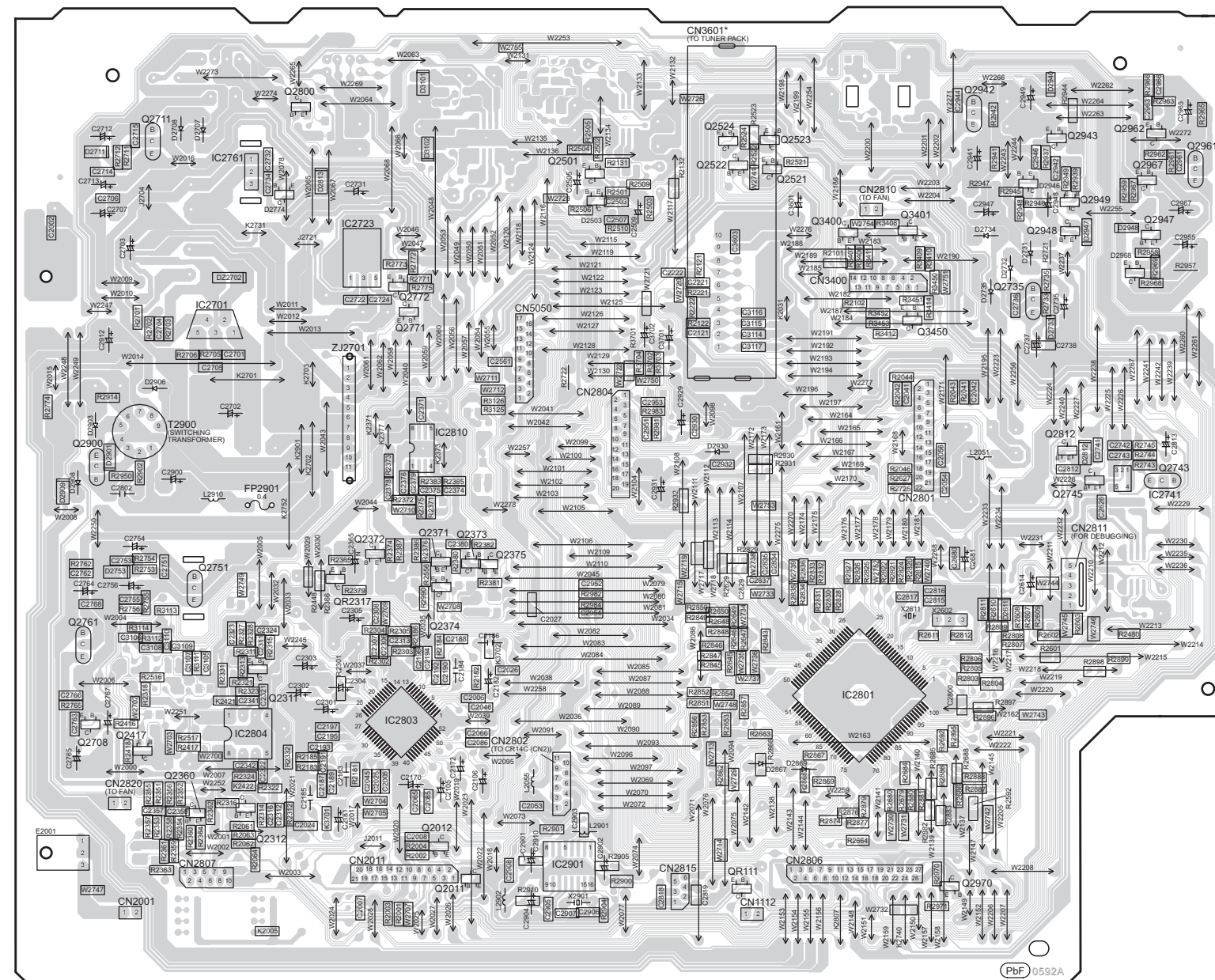
B MAIN P.C.B. (REPX0673E)
