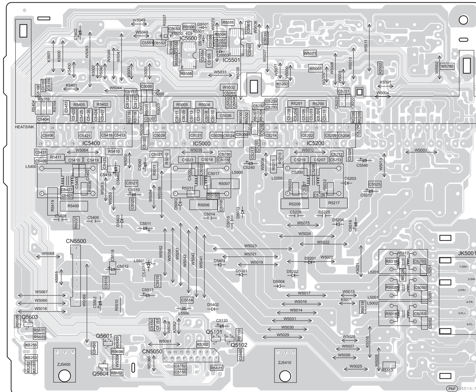
M D-AMP P.C.B (REPX0638B)
