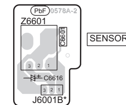
H REMOTE SENSOR P.C.B. (REPX0649C)
