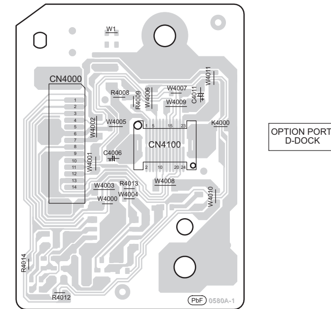
P D-PORT (OPTION PORT) P.C.B. (REPX0651A)
