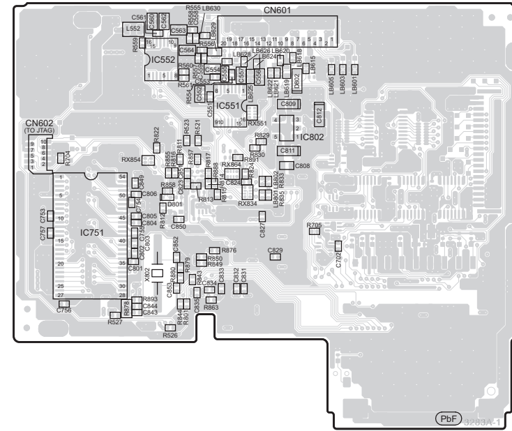
L JUPITER USB P.C.B. (REPX0660B)
