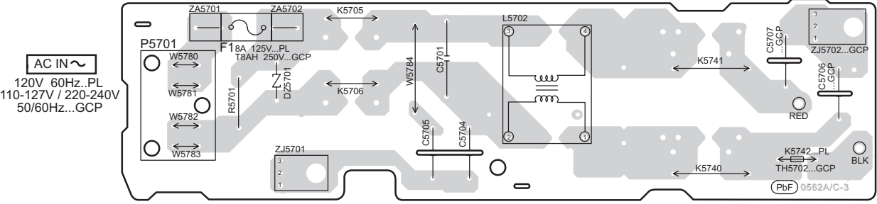
O AC INLET P.C.B. (REPX0622E...PL) (REPX0622G...GCP)
