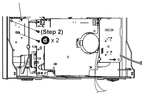
Mic P.C.B.
