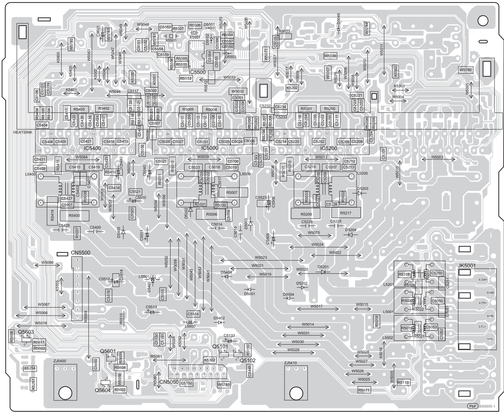
G D-AMP P.C.B. (REPX0727D)
