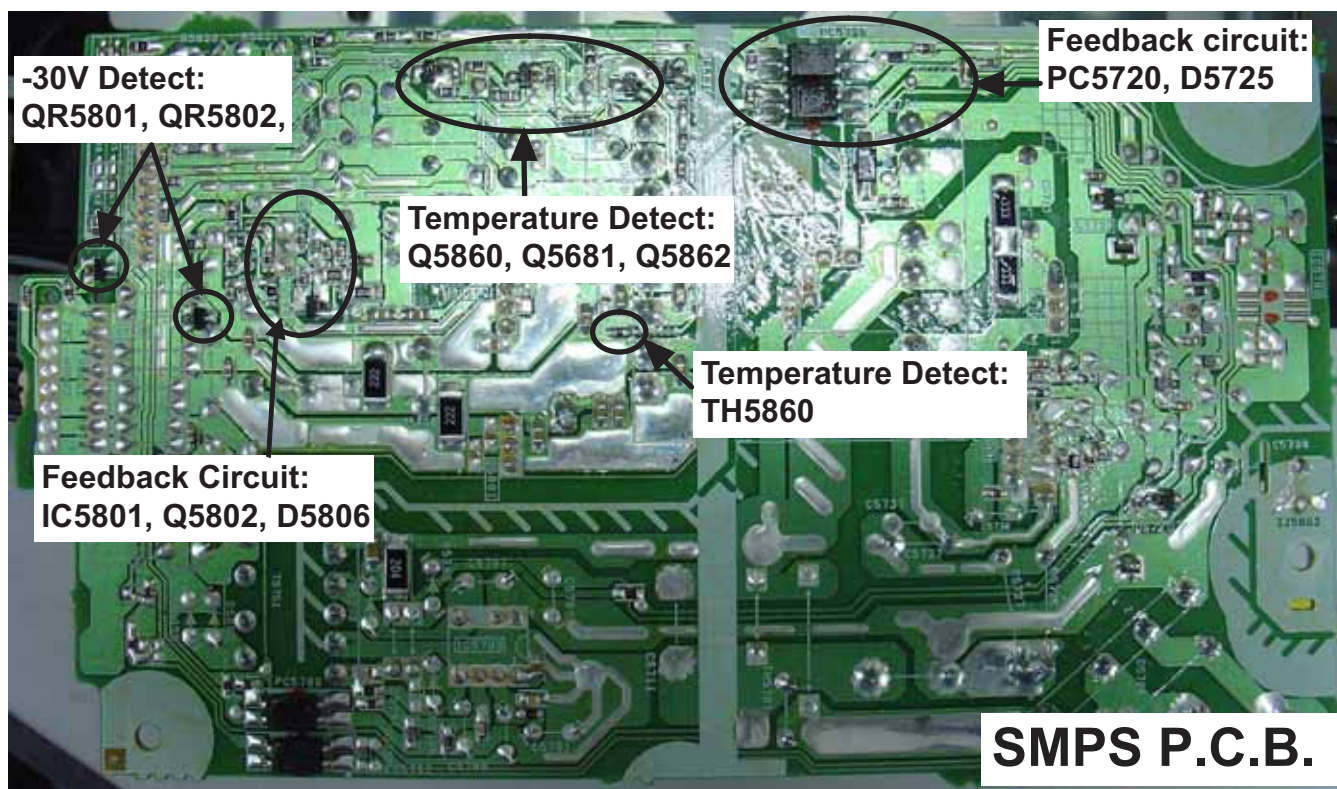
Fig. 1 SMPS P.C.B.
