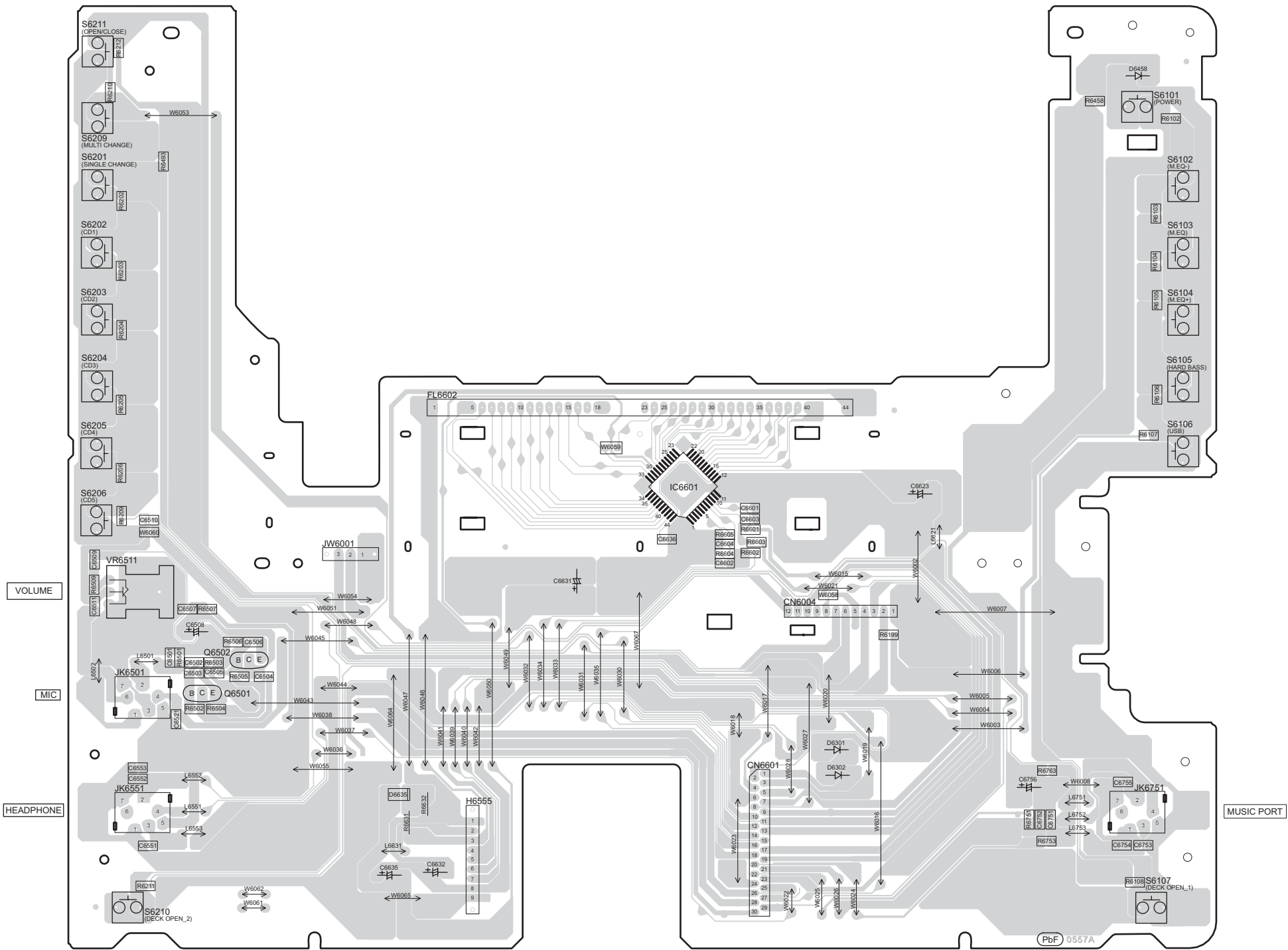
C PANEL P.C.B (REPX0612A)
