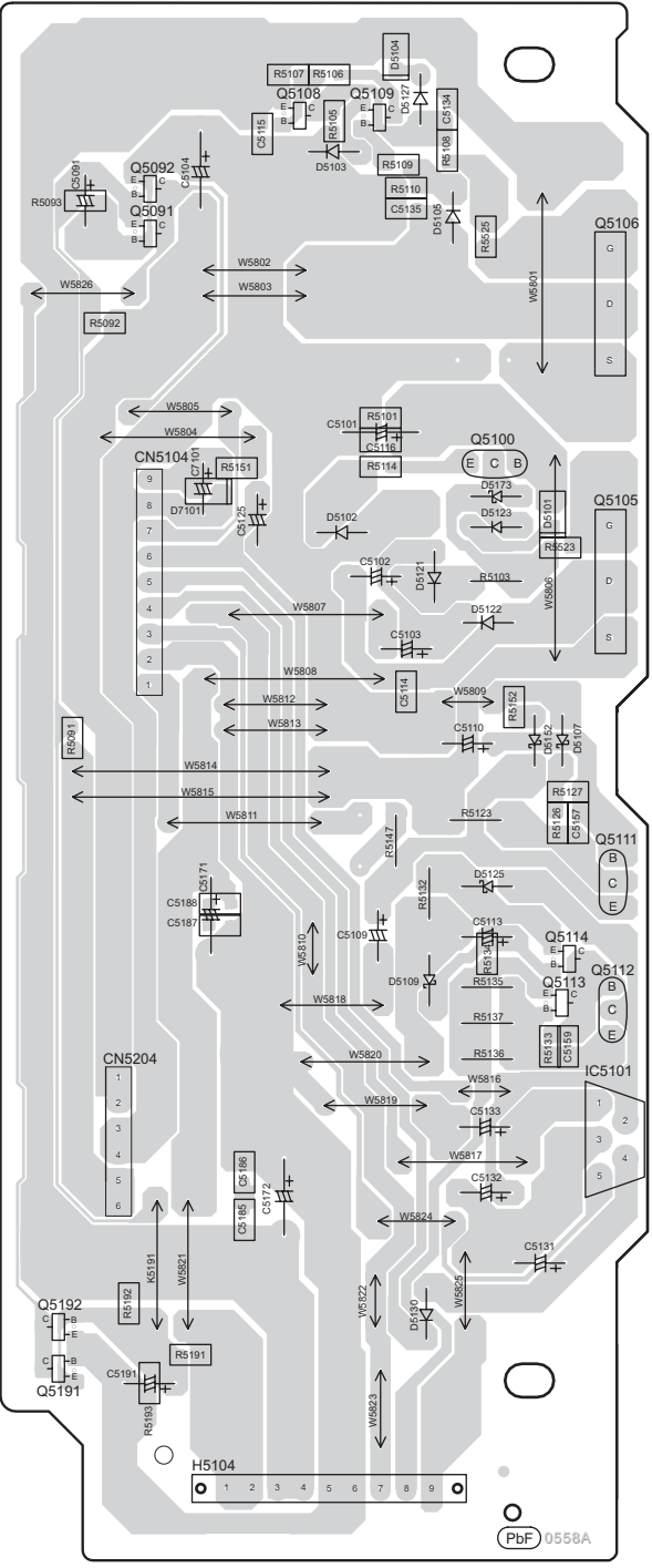
I SUB POWER P.C.B (REPX0613A)
