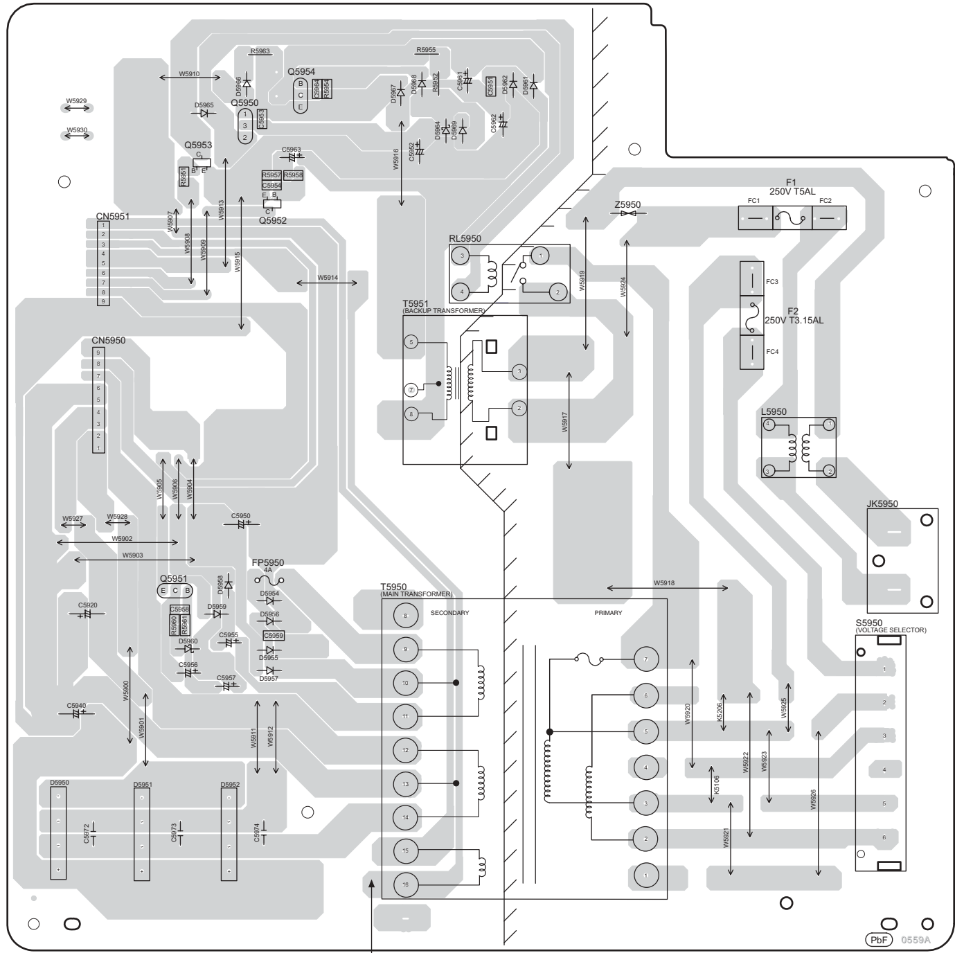
L TRANSFORMER P.C.B (REPX0614A)
