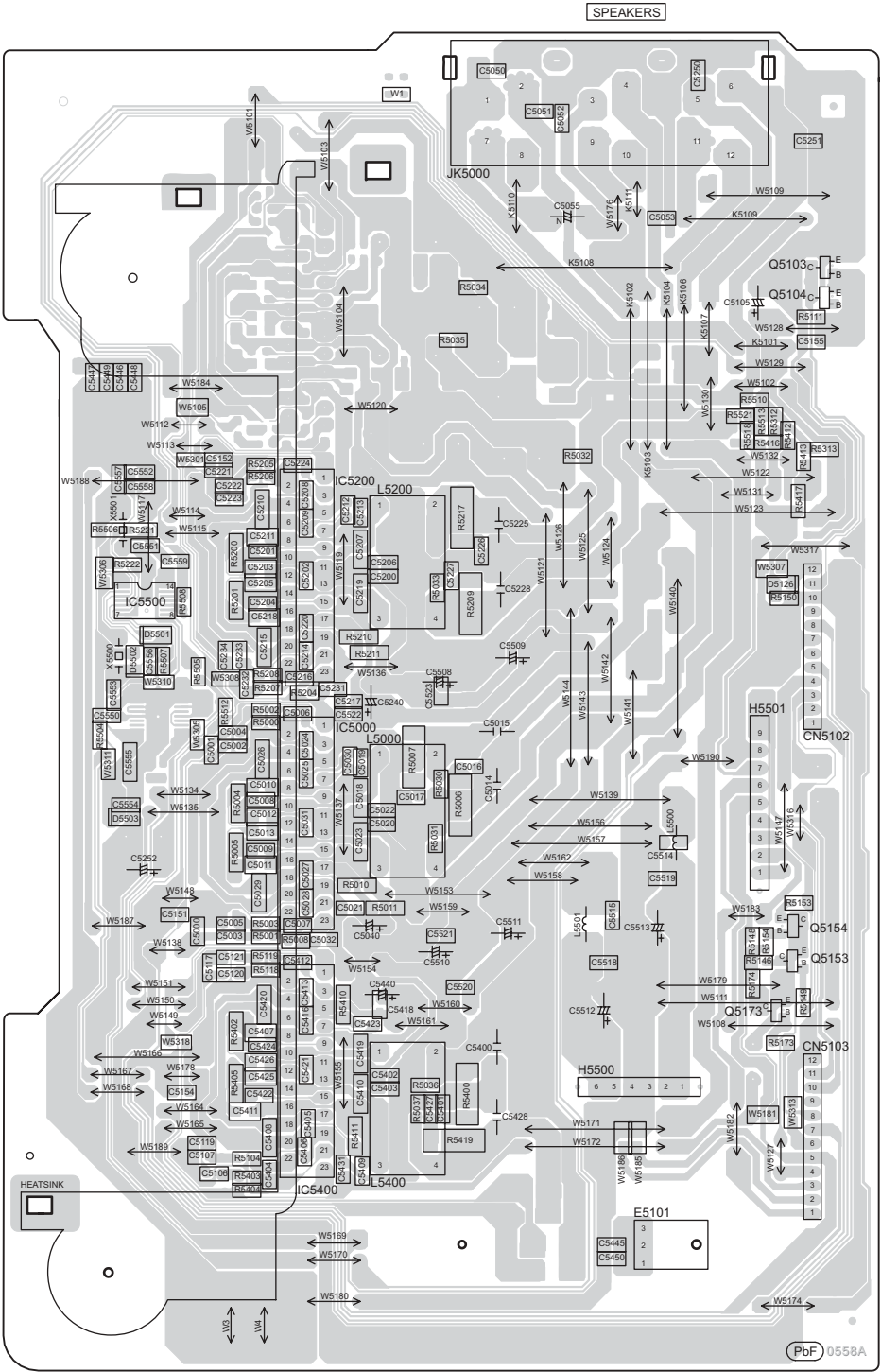
H POWER P.C.B (REPX0613A)
