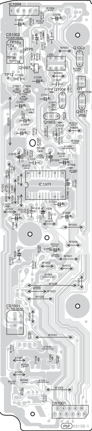
J DECK P.C.B (REPX0618A)
