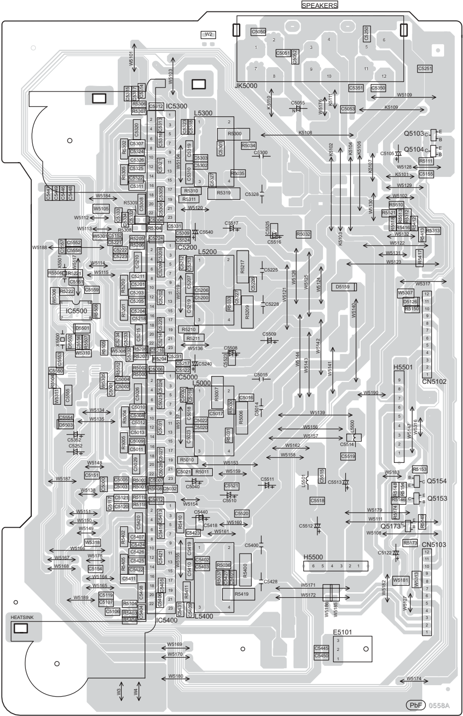
H POWER P.C.B (REPX0609A)
