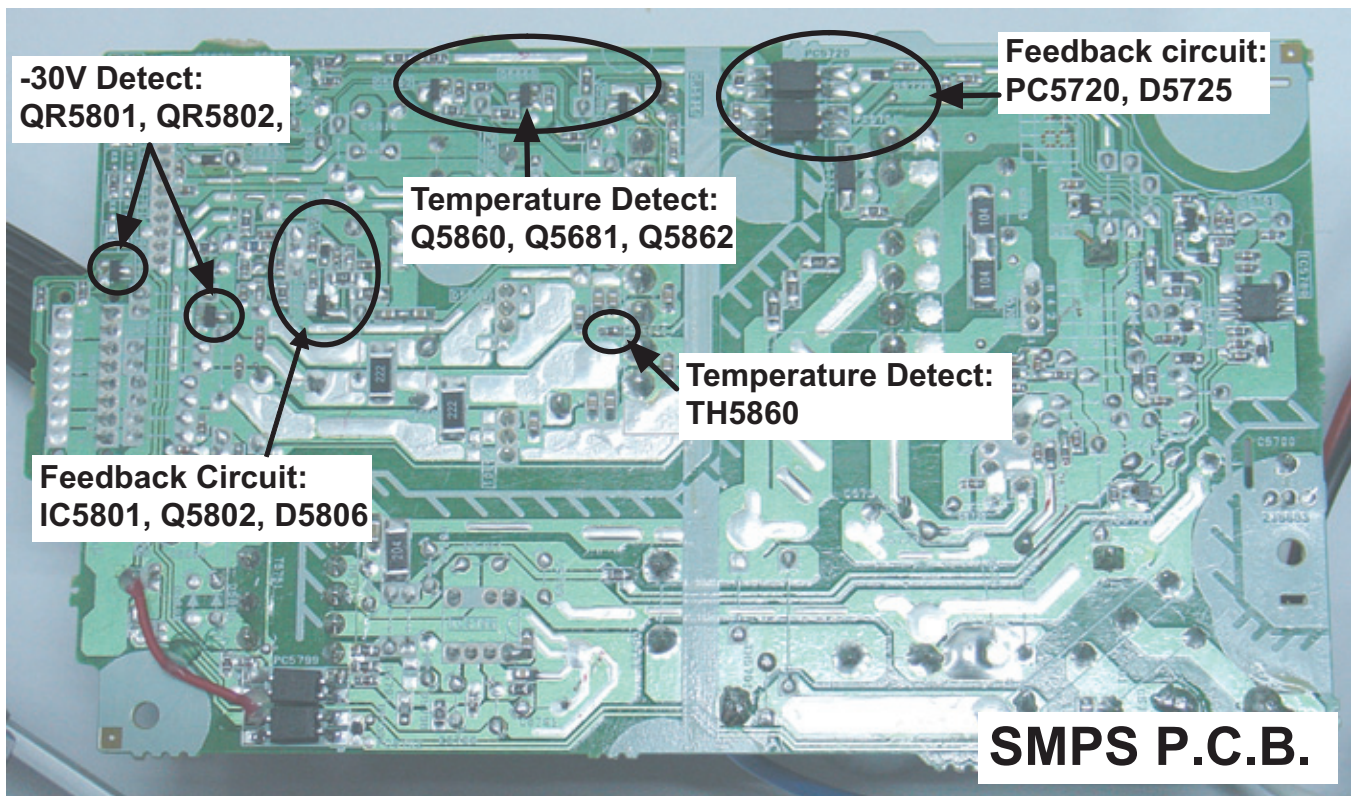
Fig. 1 SMPS P.C.B.
