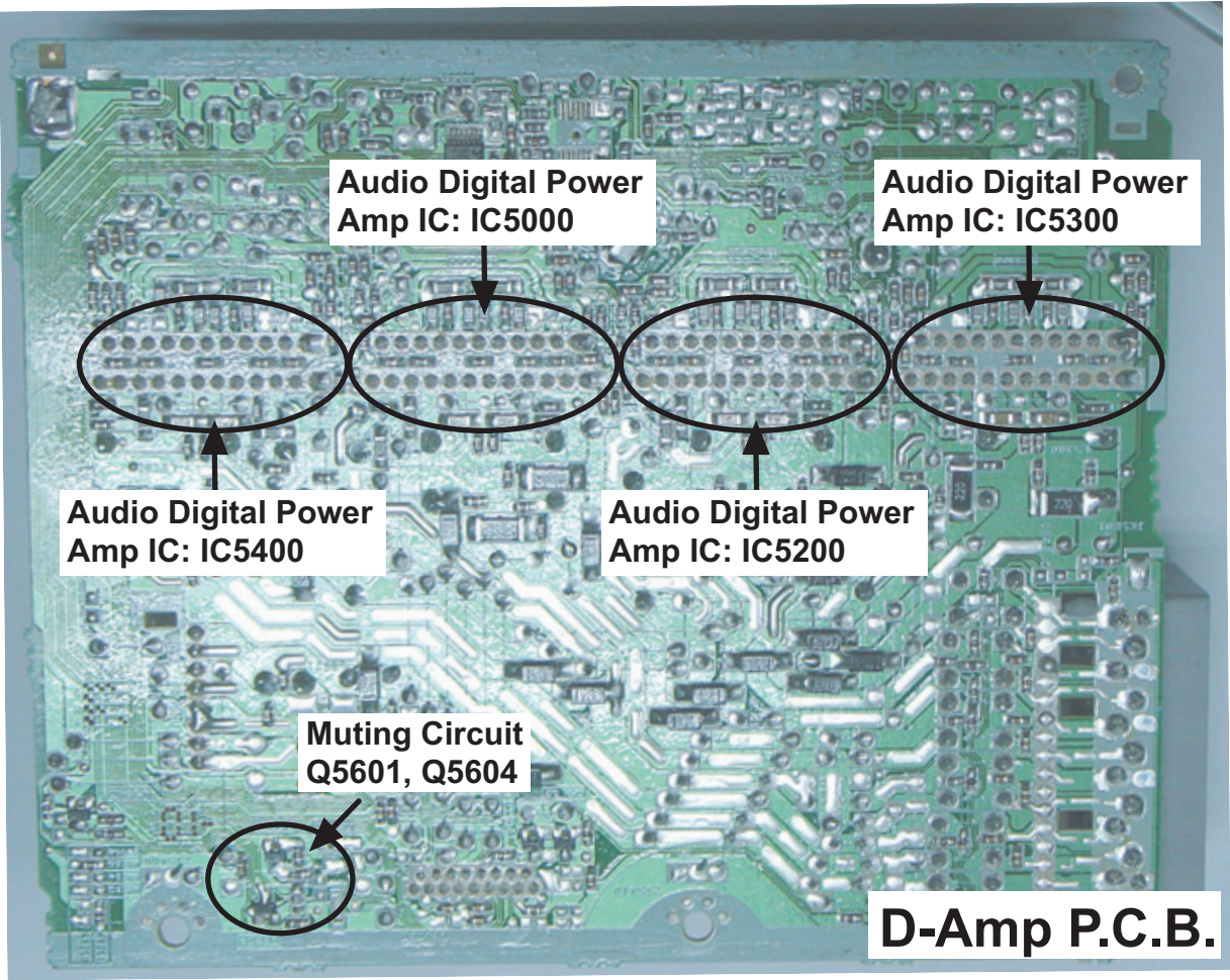
Fig. 2 D-Amp P.C.B.
