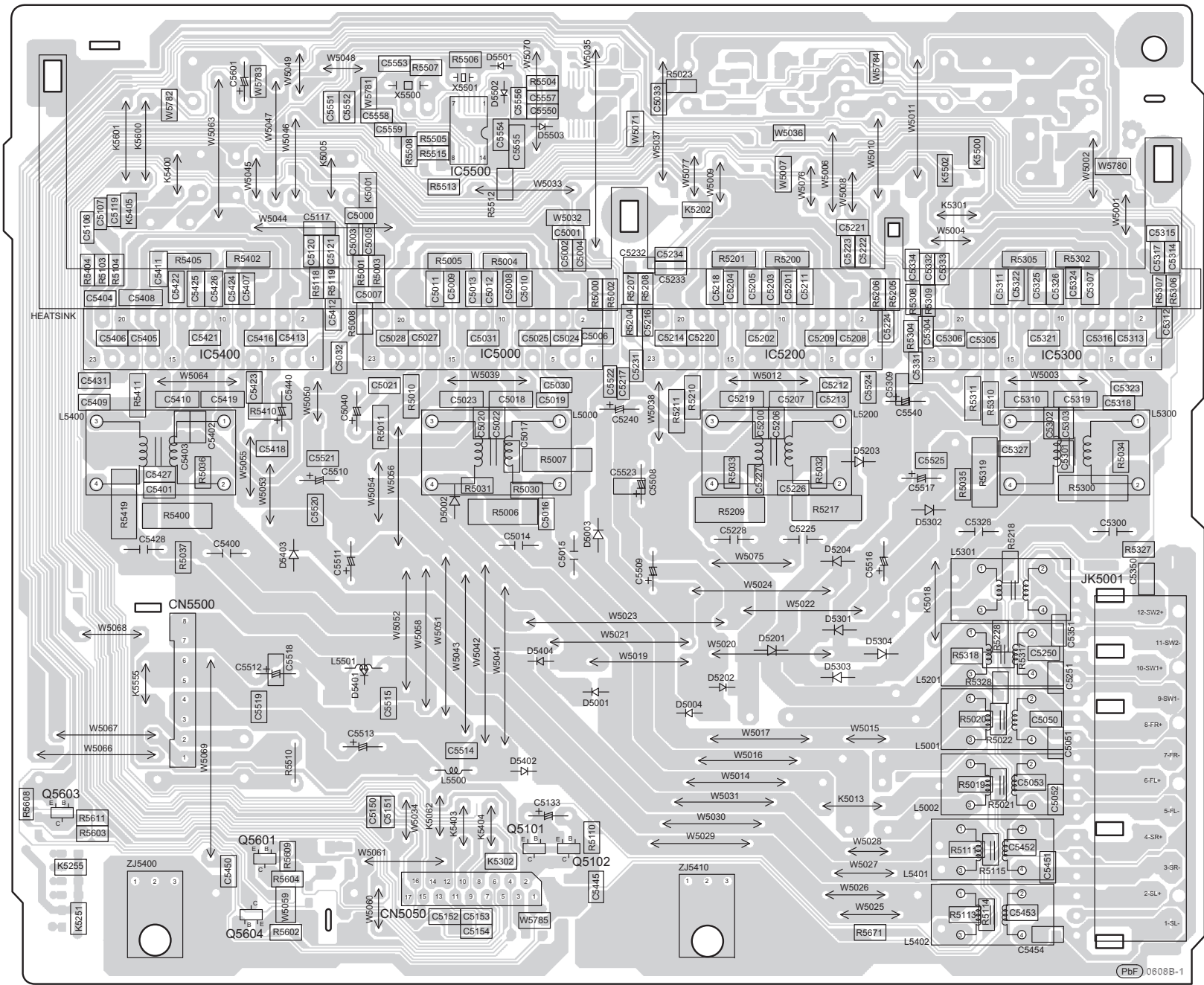
G D-AMP P.C.B. (REPX0727E)
