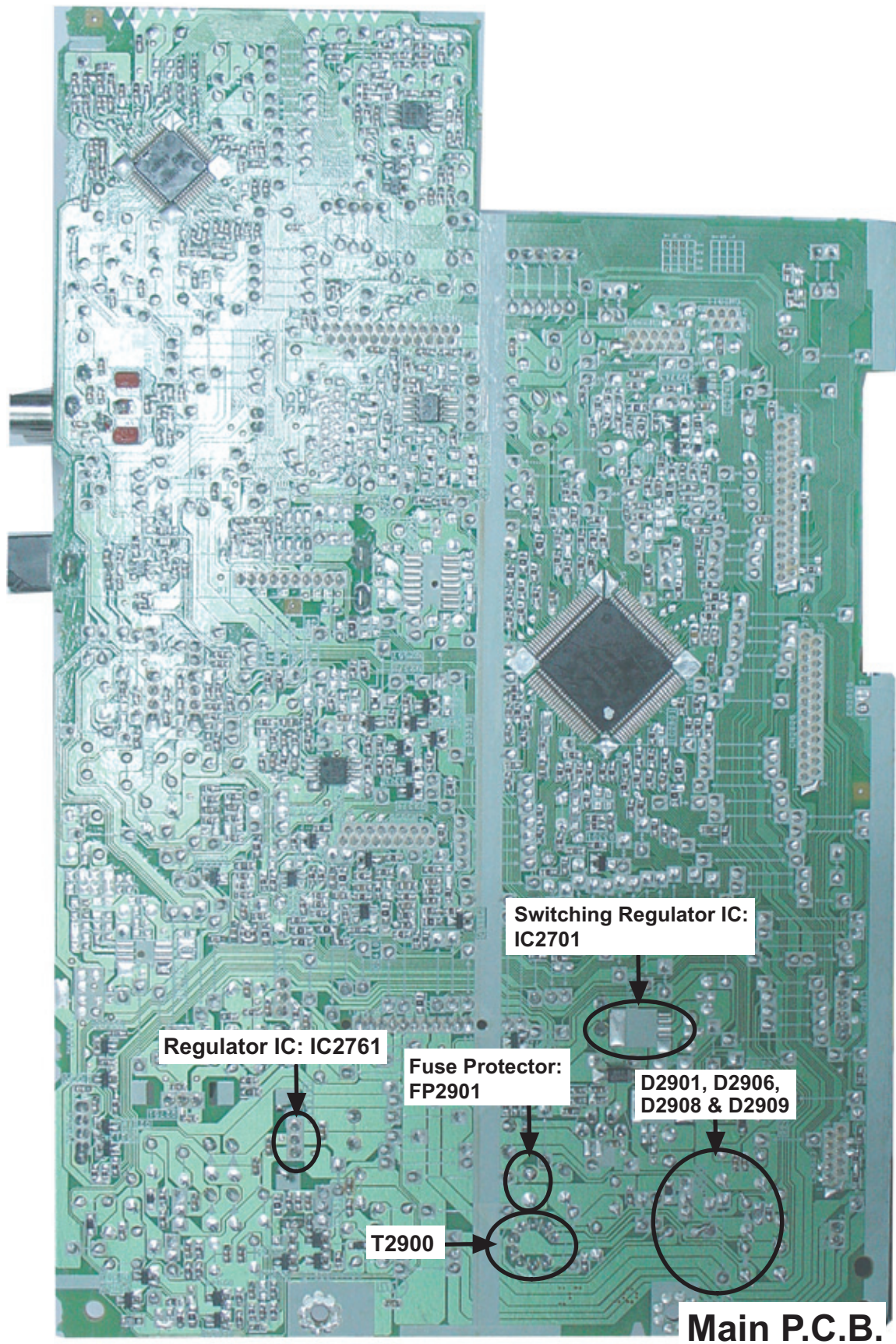
Fig. 3 Main P.C.B.
