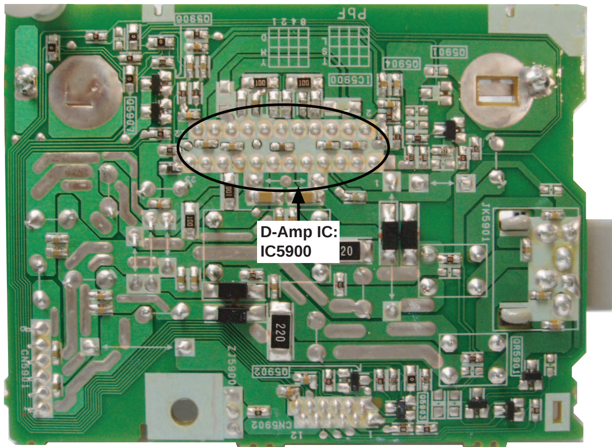
Fig. 3 D-Amp P.C.B.
