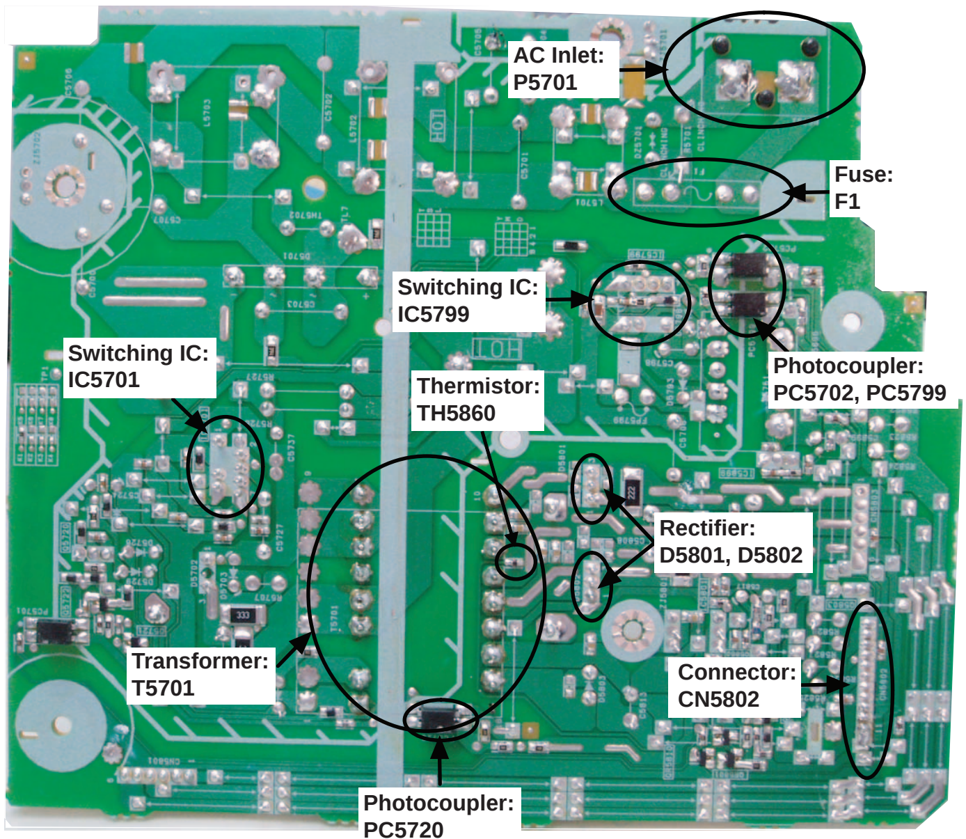
Fig. 1 SMPS P.C.B.
