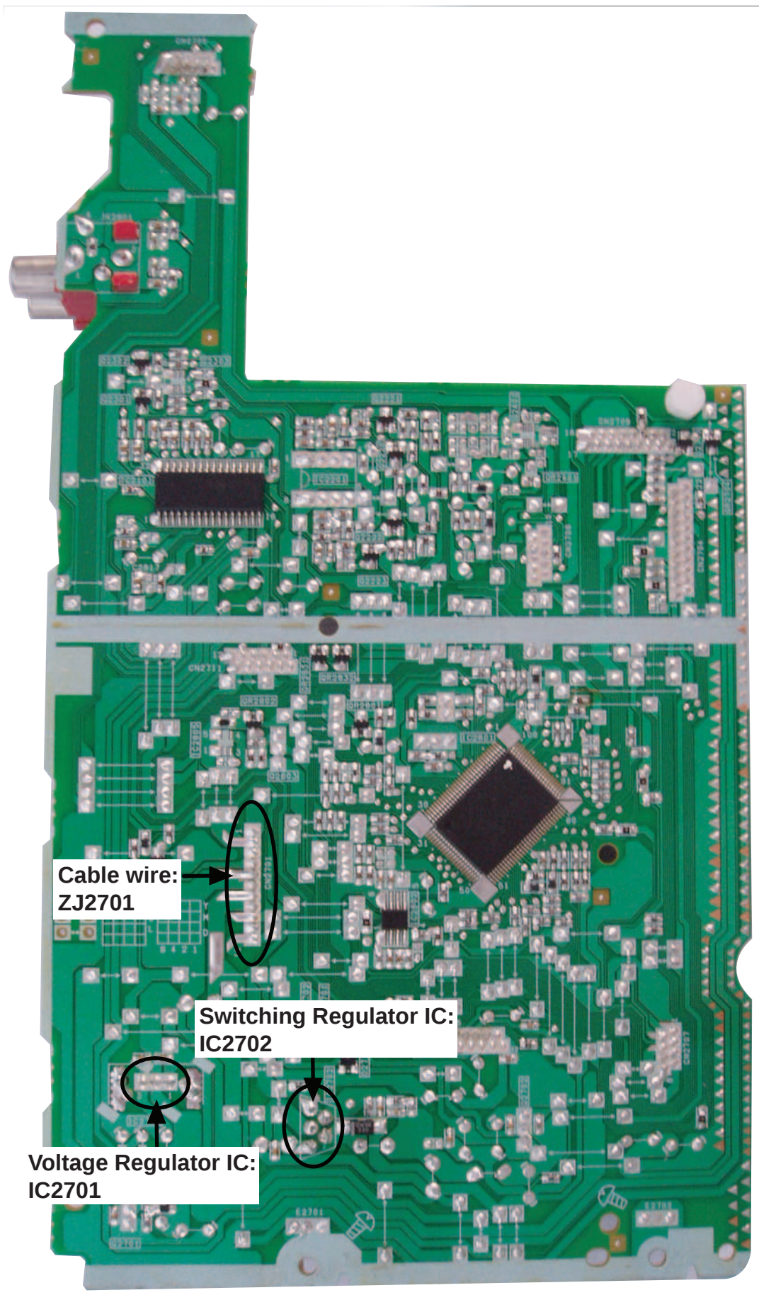
Fig. 2 Main P.C.B.
