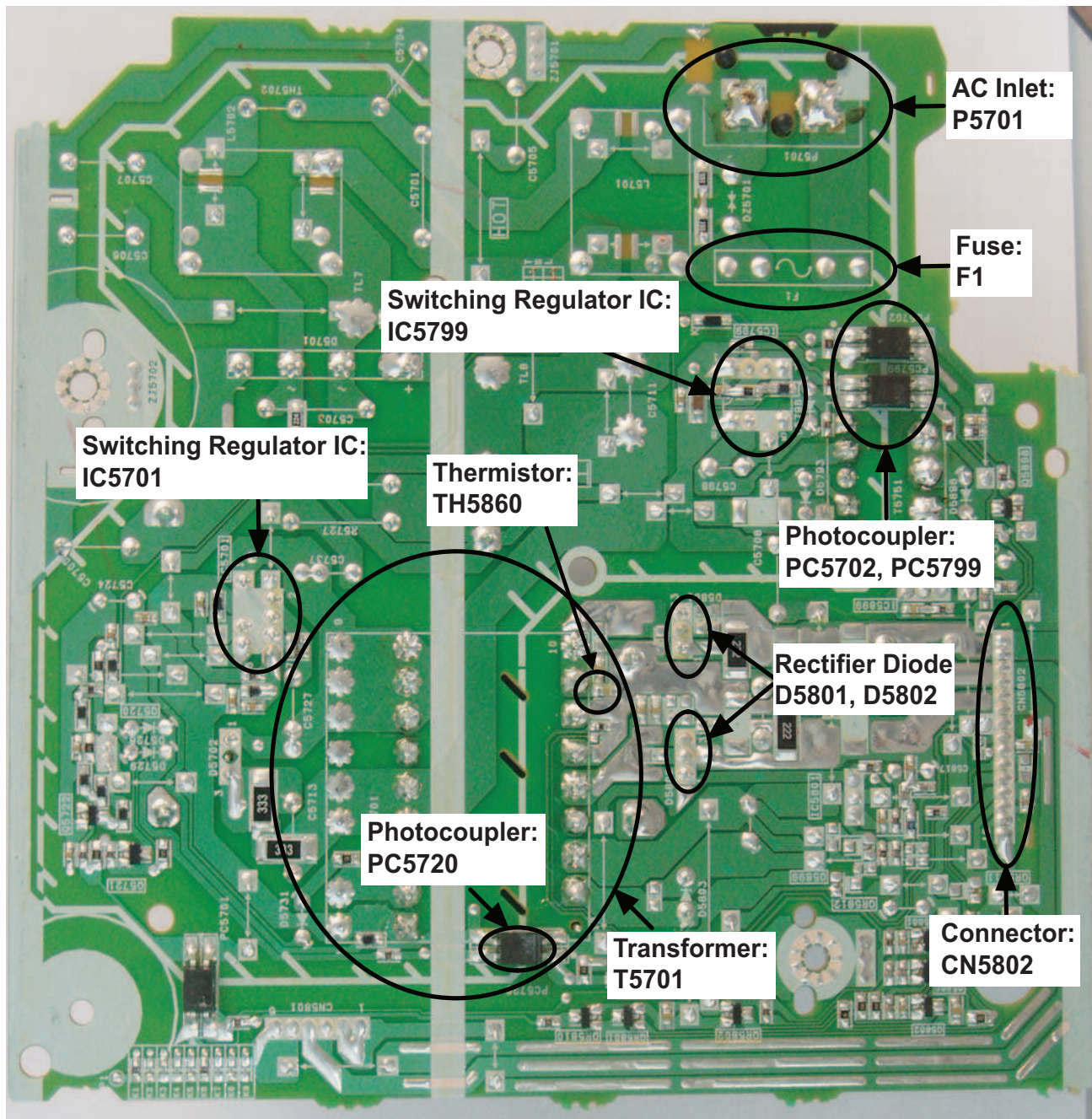
Fig. 1 SMPS P.C.B.
