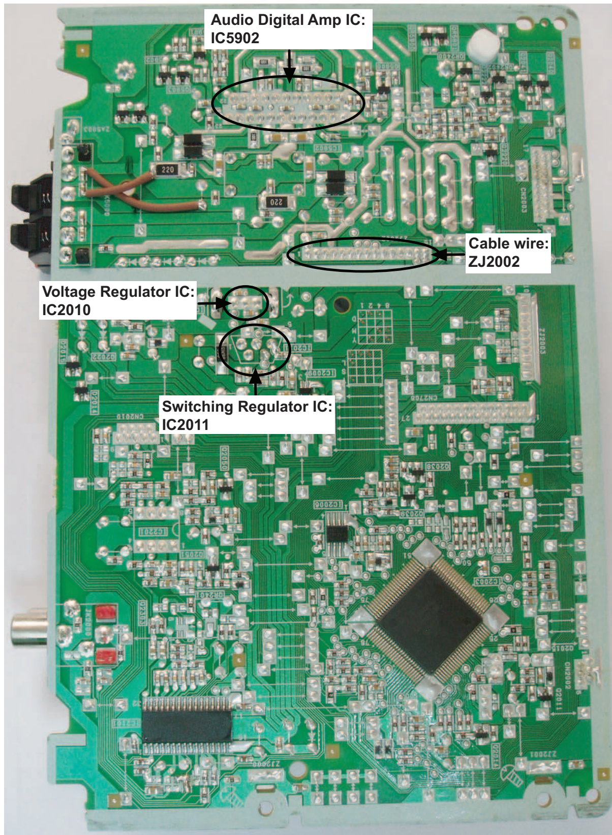
Fig. 2 Main P.C.B.
