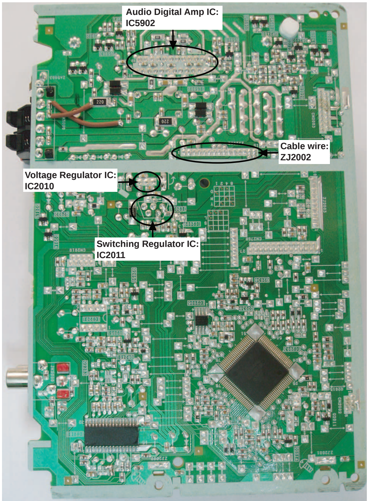
Fig. 2 Main P.C.B.
