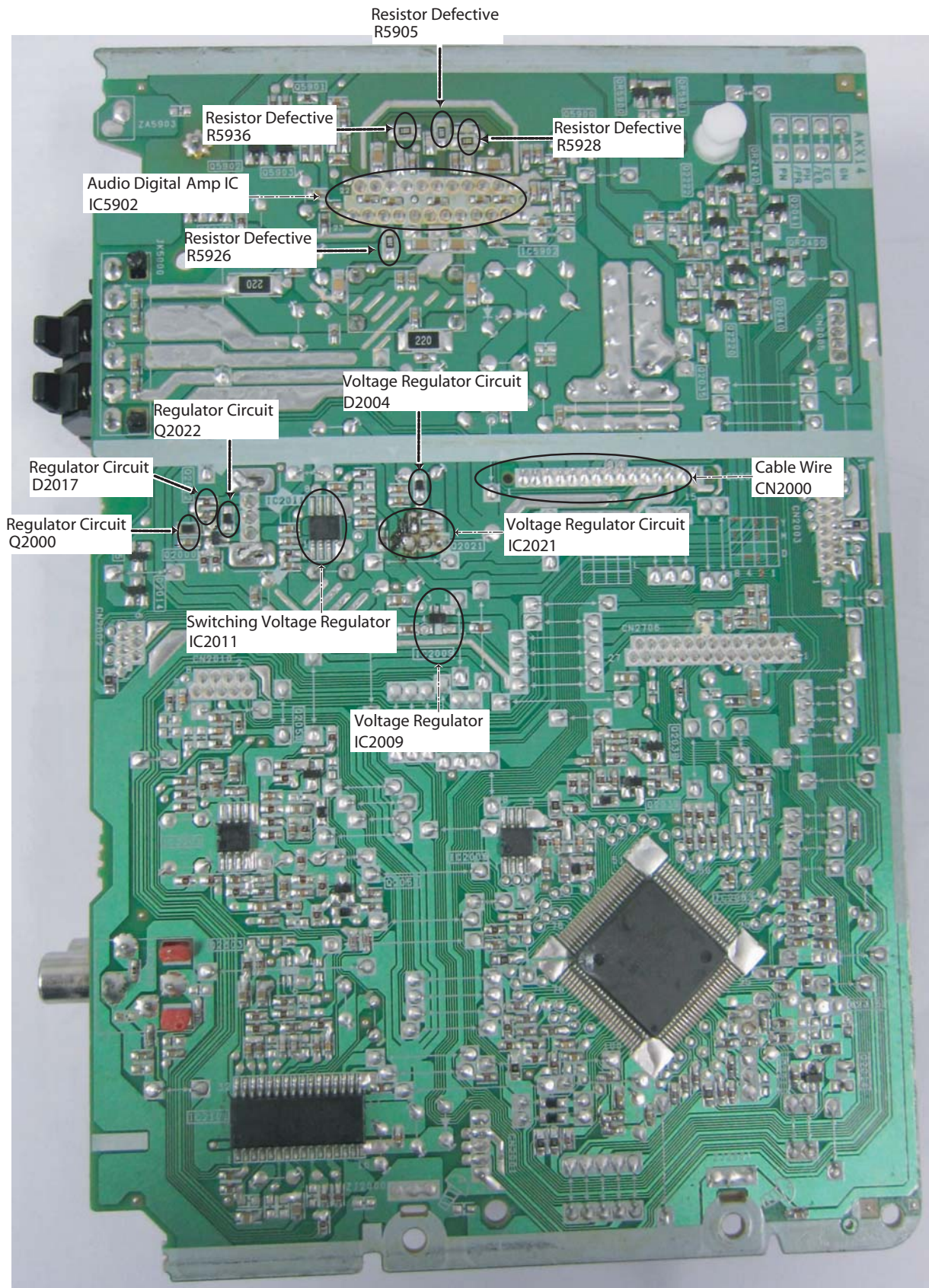
Fig. 2 Main P.C.B.
