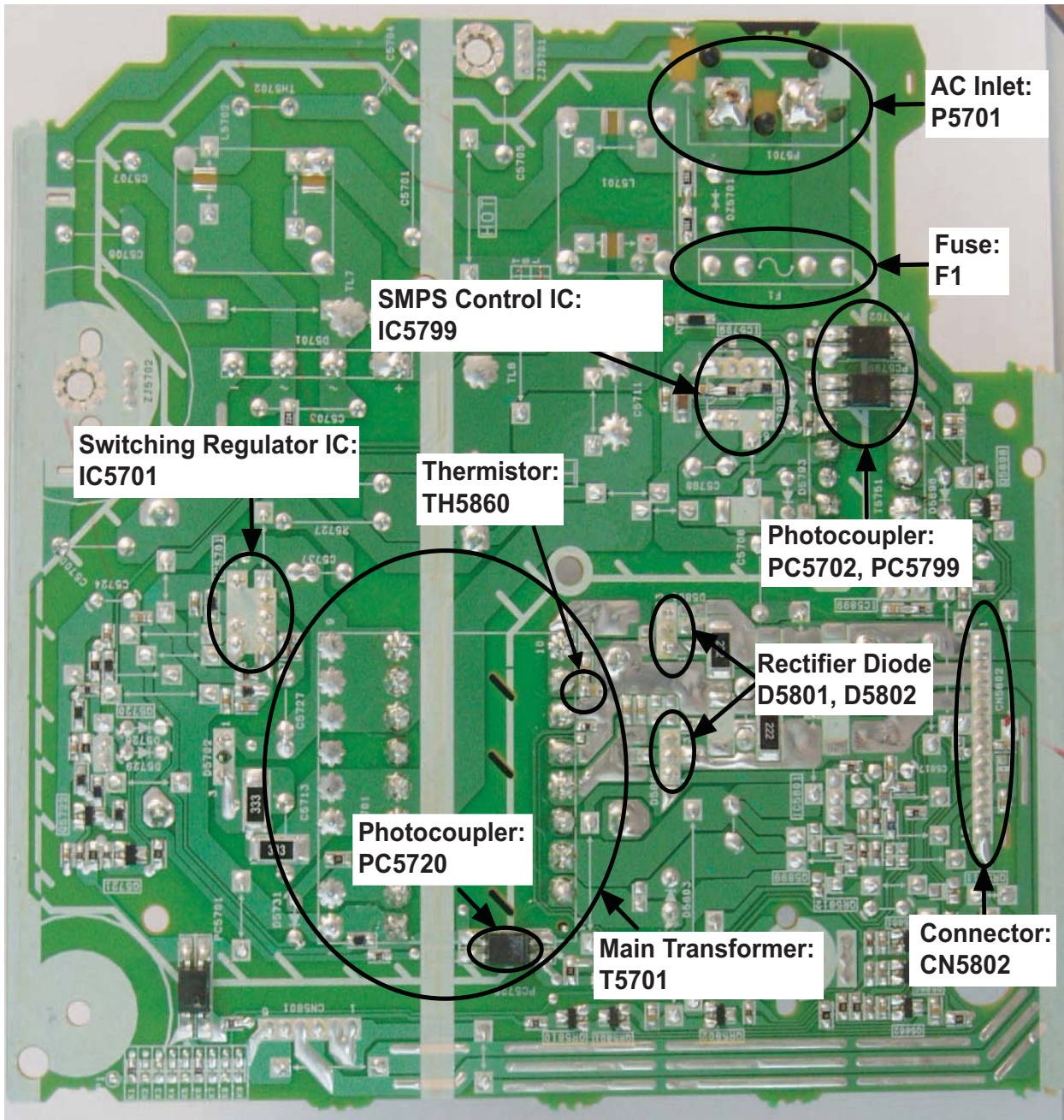
Fig. 1 SMPS P.C.B.
