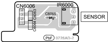
E REMOTE SENSOR P.C.B. (REPX0887KD...PH) (REPX0887HD...PN)
