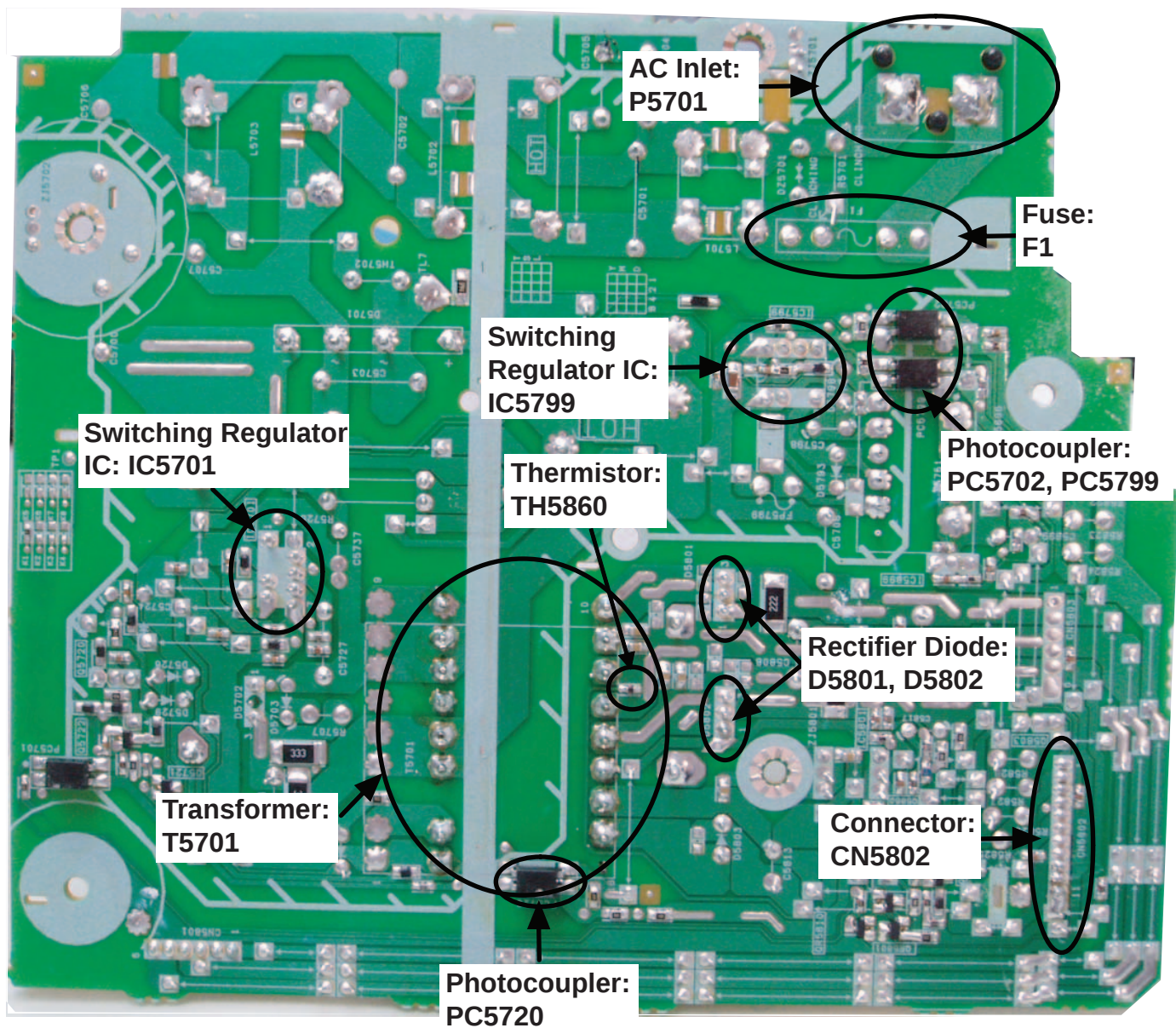
Fig. 1 SMPS P.C.B.
