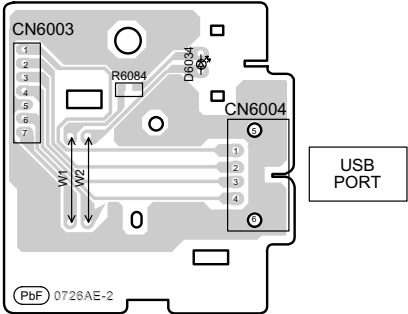
F USB P.C.B. (REPX0887KE...PH) (REPX0887HE...PN)
