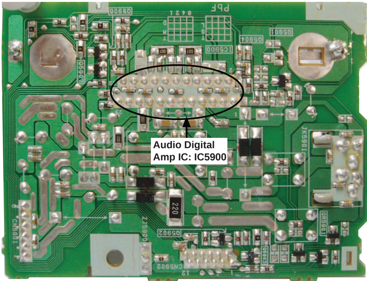
Fig. 3 D-Amp P.C.B.
