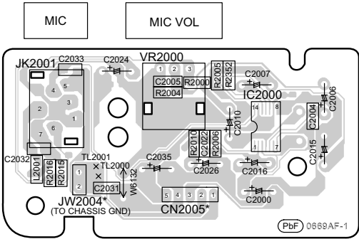
K MIC P.C.B. (REPX0815FF...PH) (REPX0815DF...PN)
