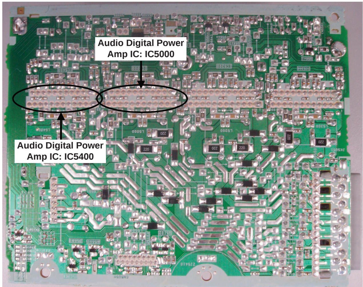
Fig. 3 D-Amp P.C.B.
