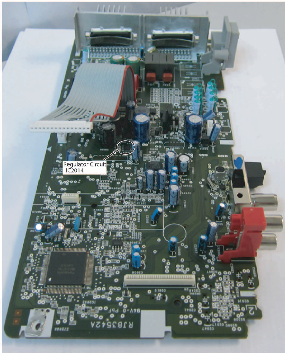
Fig. 2 Main P.C.B.
