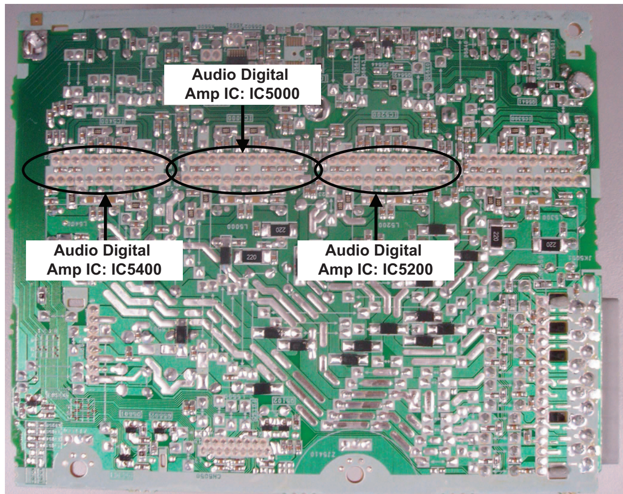
Fig. 3 D-Amp P.C.B.
