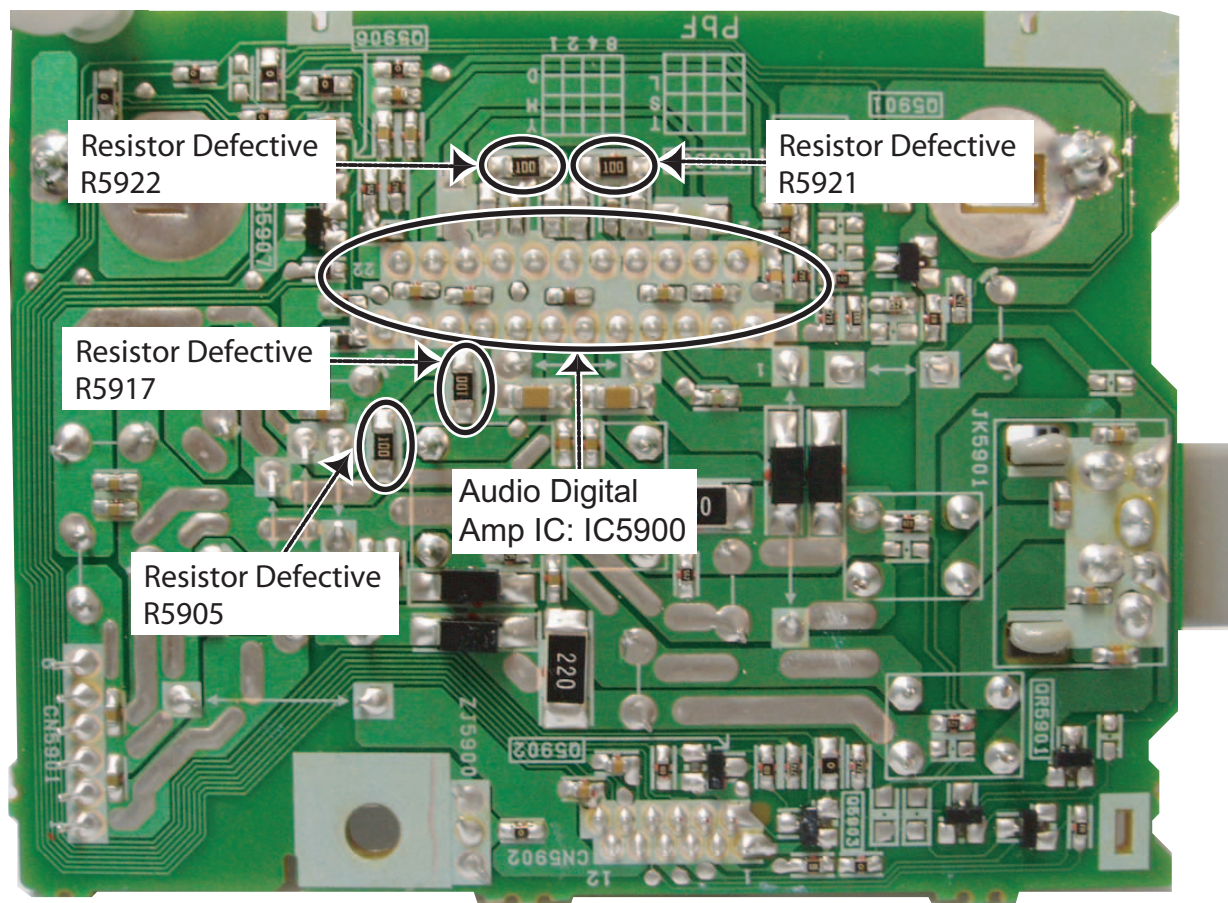
Fig. 4 D-Amp P.C.B.
