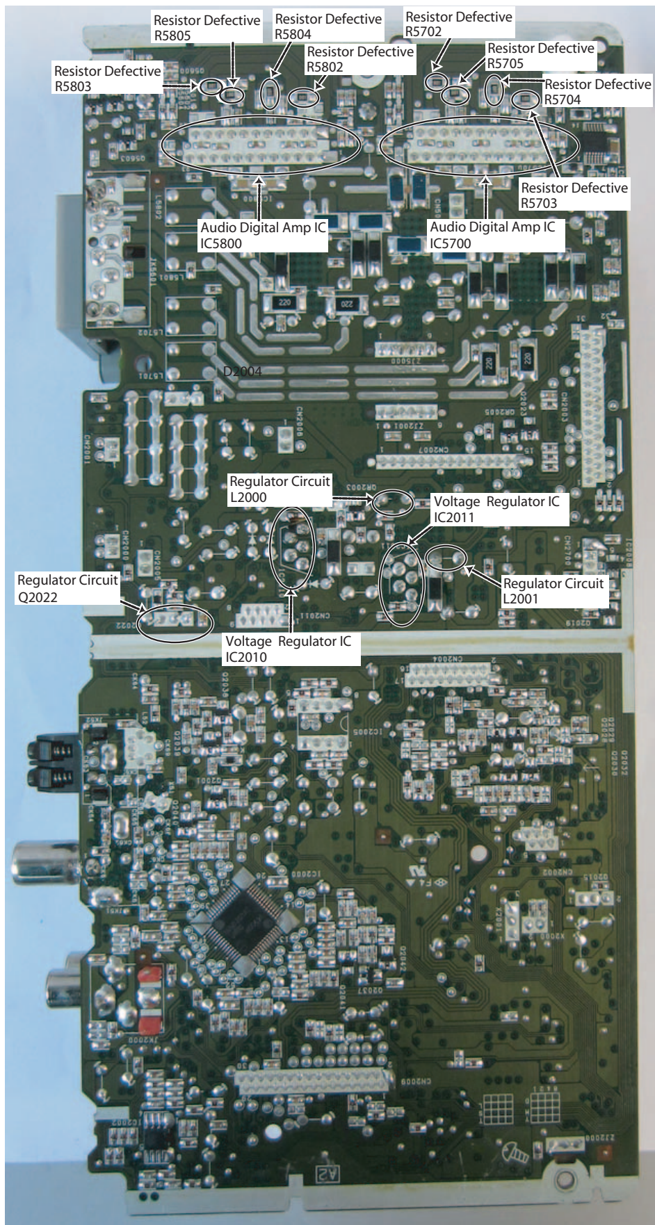
Fig. 3 Main P.C.B. (Back Side)
