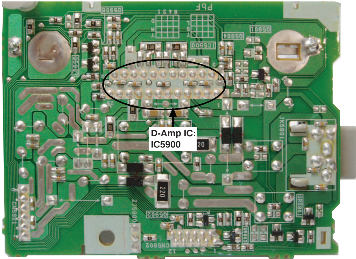
Fig. 4 Surround D-Amp P.C.B.
