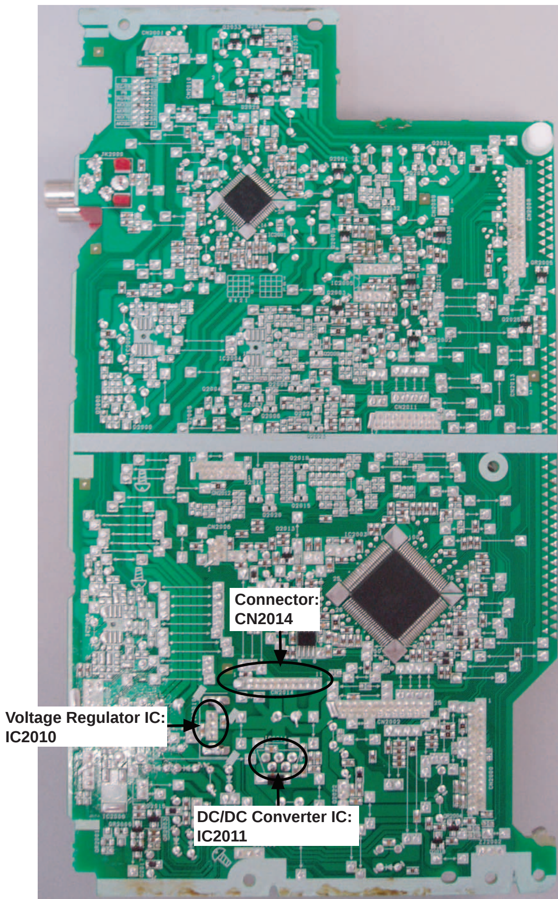
Fig. 2 Main P.C.B.
