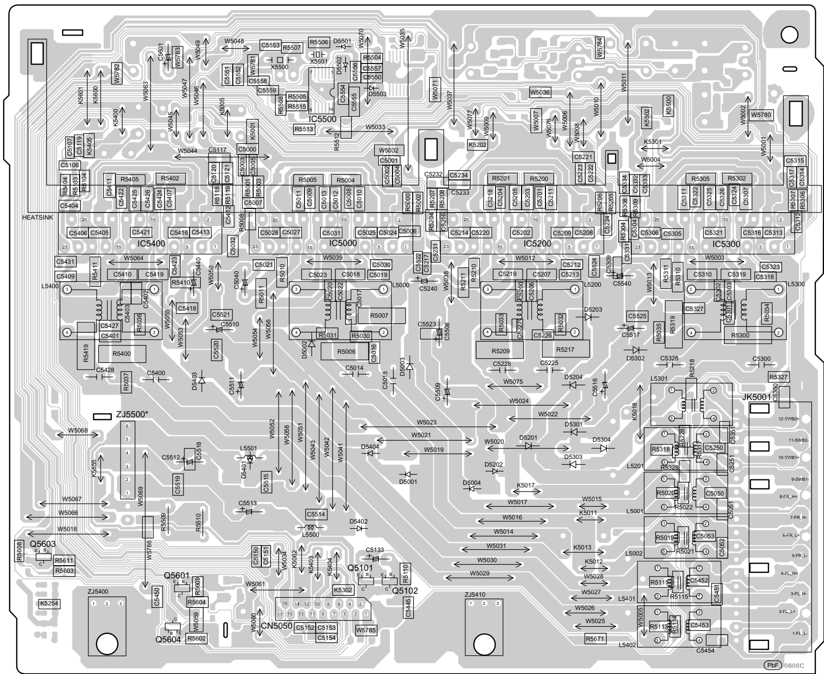
I D-AMP P.C.B. (REPX0821D)
