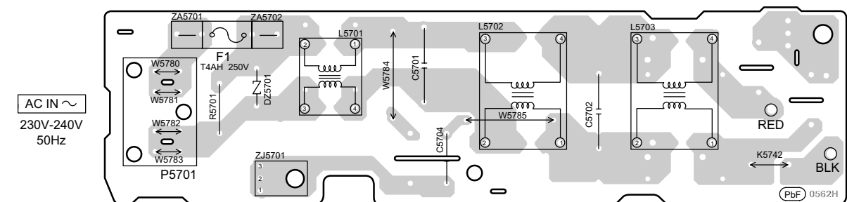
M AC INLET P.C.B. (REPX0622W)
