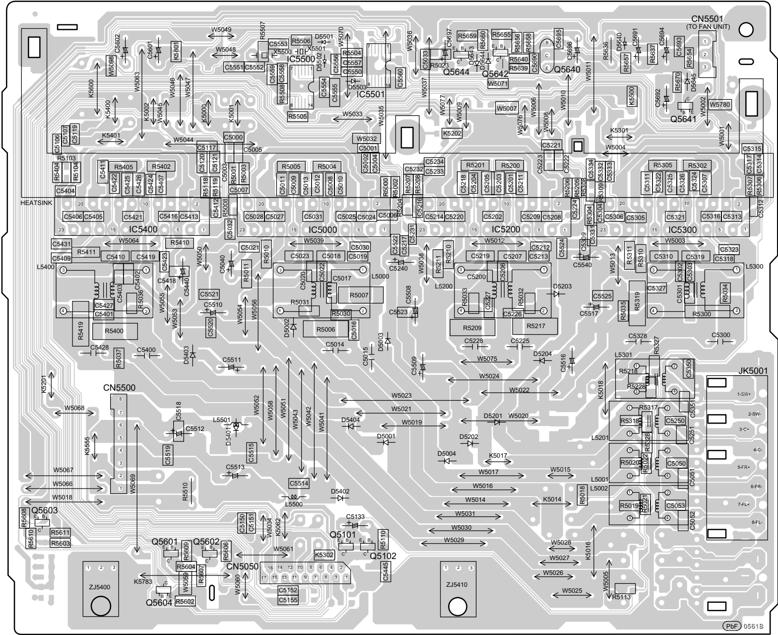
K D-AMP P.C.B. (REPX0621G)
