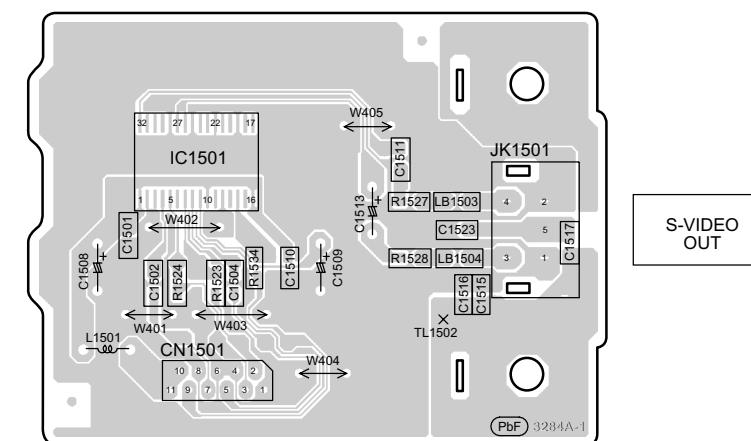
N S-VIDEO P.C.B. (REP4371B)
