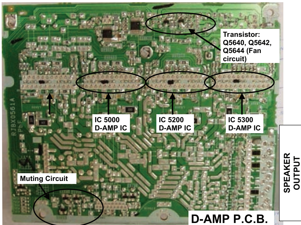
Fig. 2 D-AMP P.C.B.
