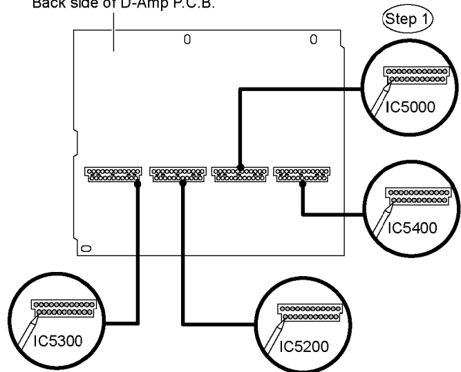
Back side of D-Amp P.C.B.
