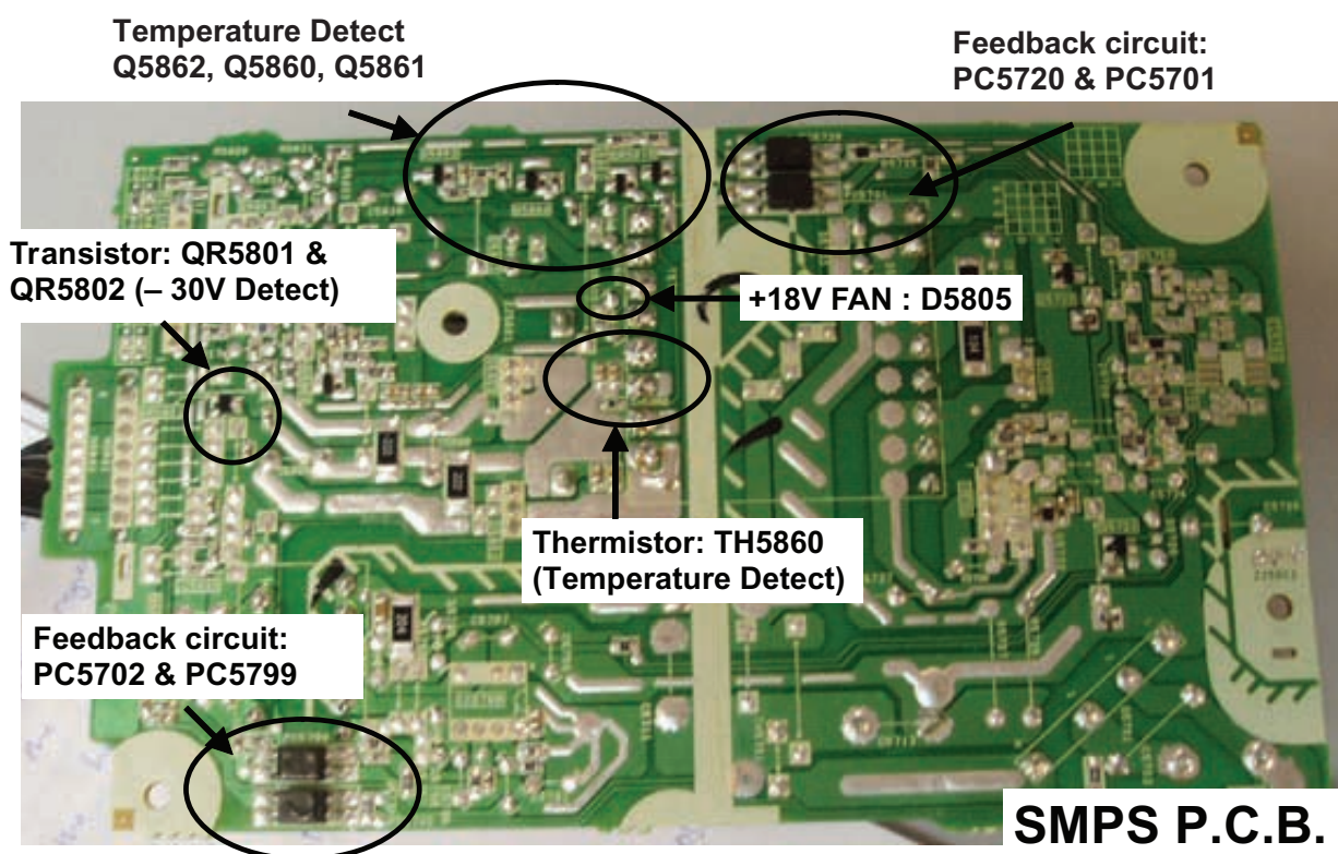
Fig. 1 SMPS P.C.B.
