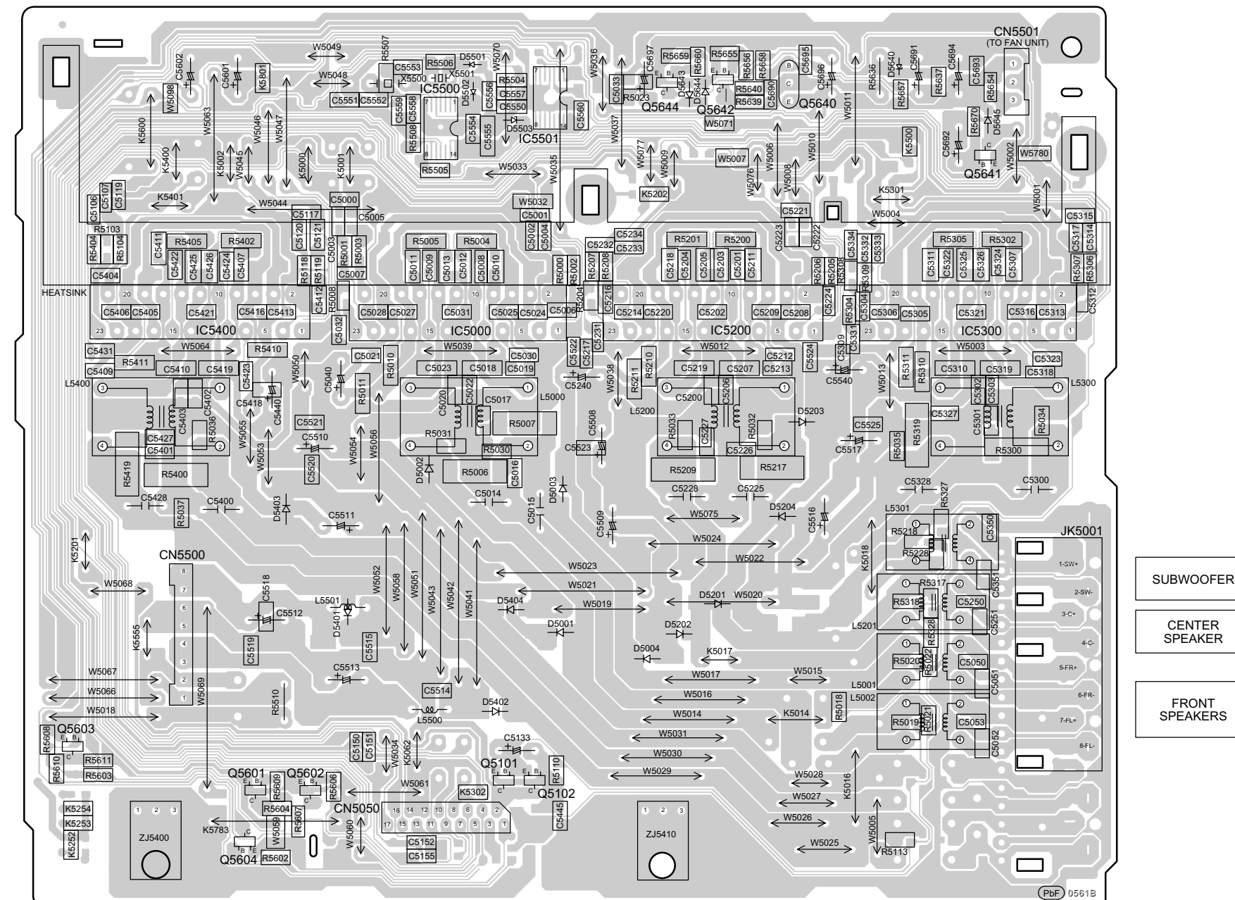
K D-AMP P.C.B. (REPX0621G)
