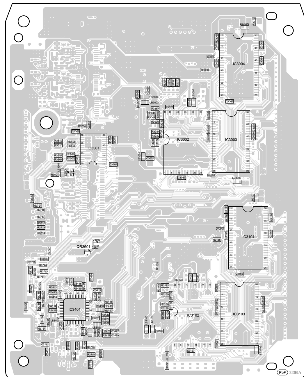
B DSP P.C.B. (REP4369A)
