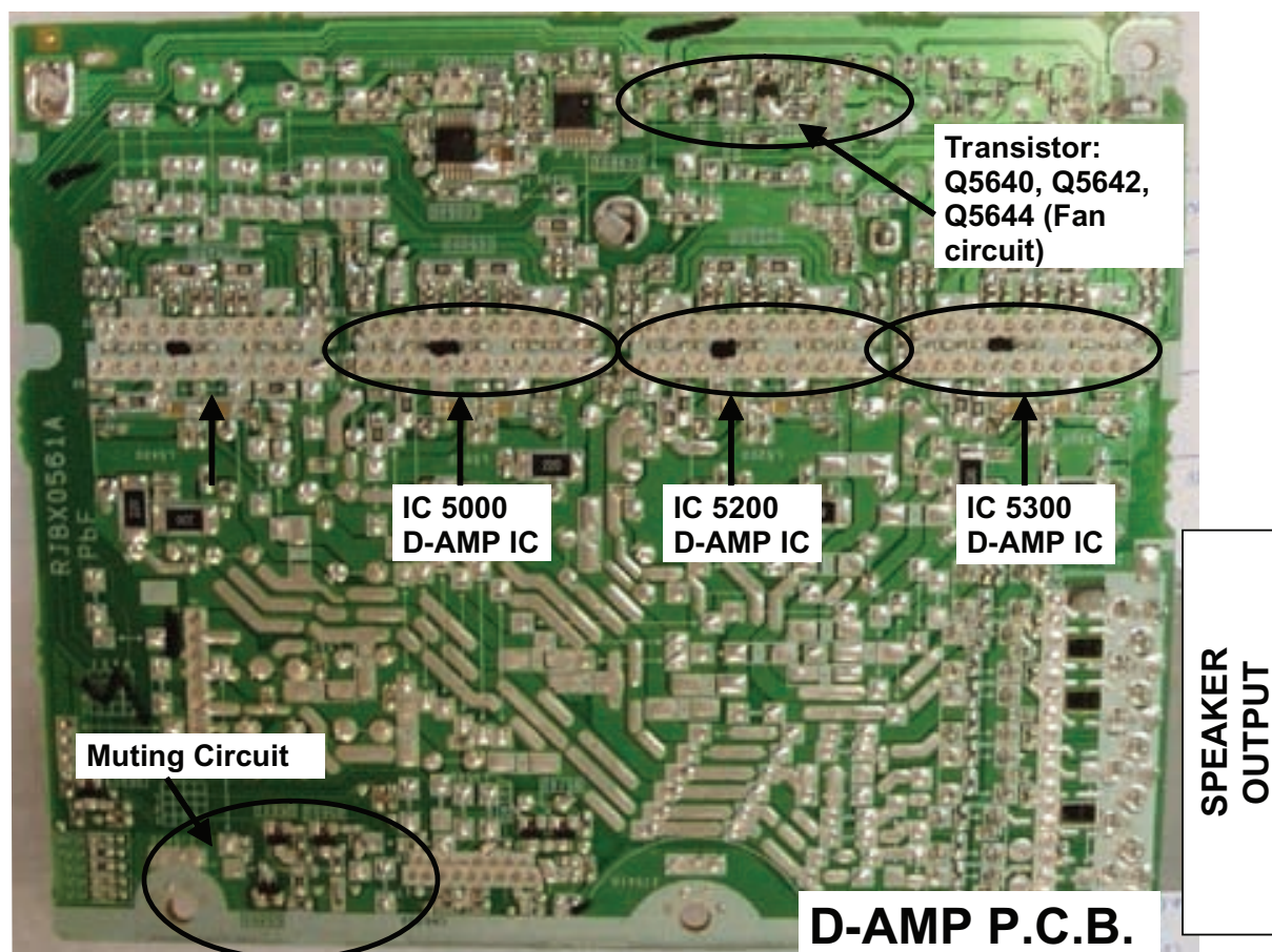
Fig. 2 D-AMP P.C.B.
