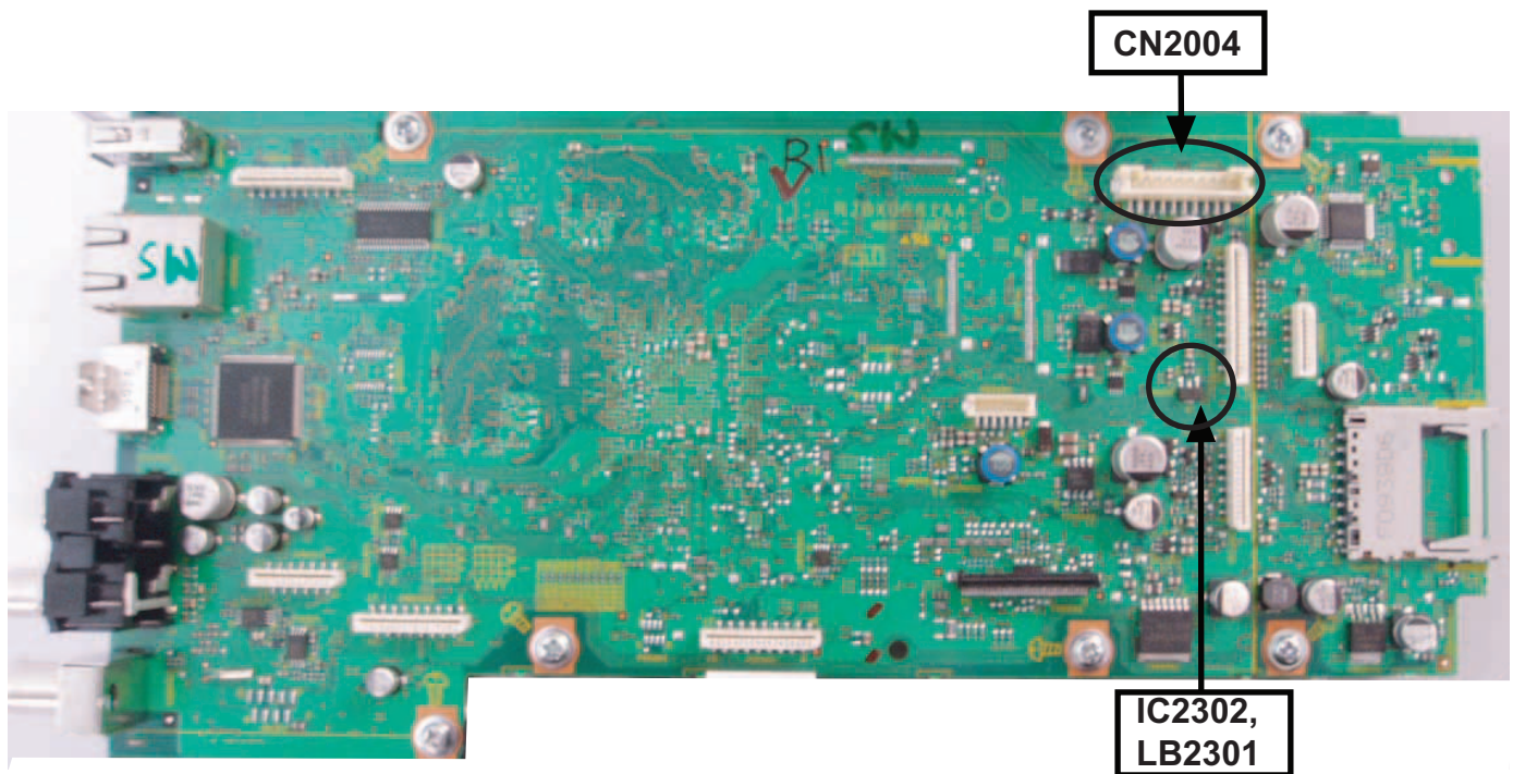
Fig 3. Main P.C.B.
