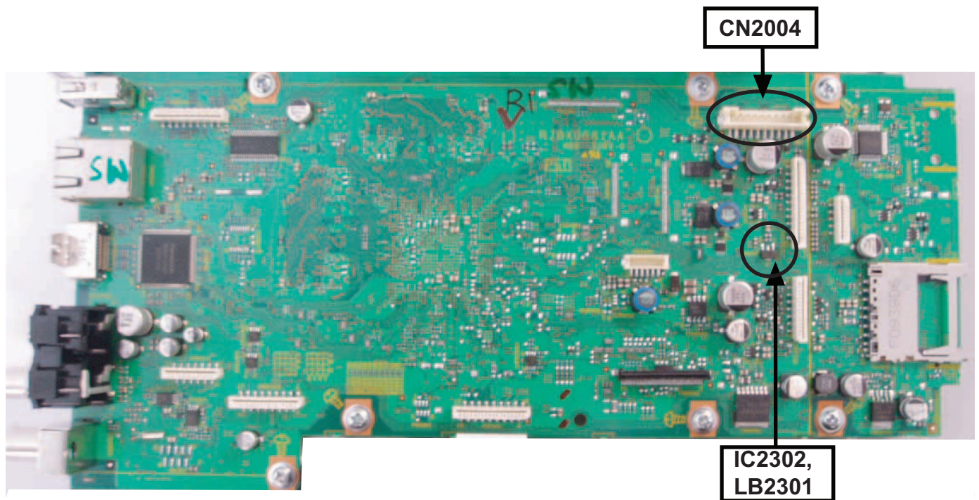
Fig 3. Main P.C.B.
