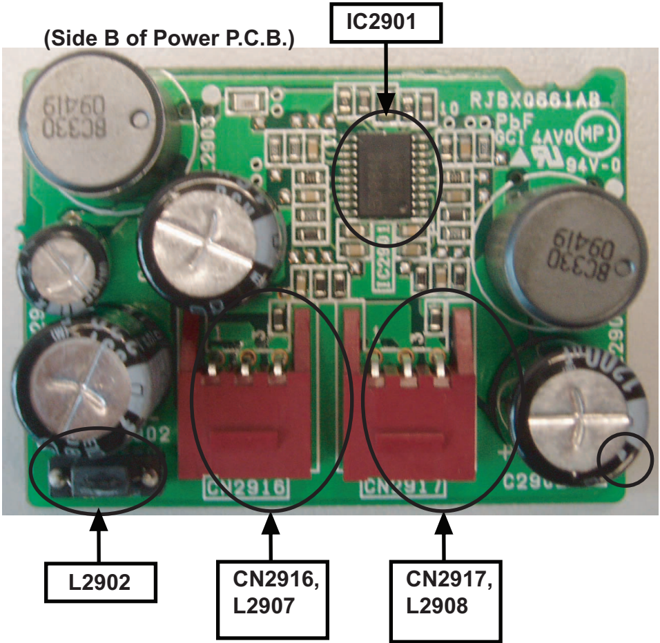
Fig 2. Power P.C.B.
