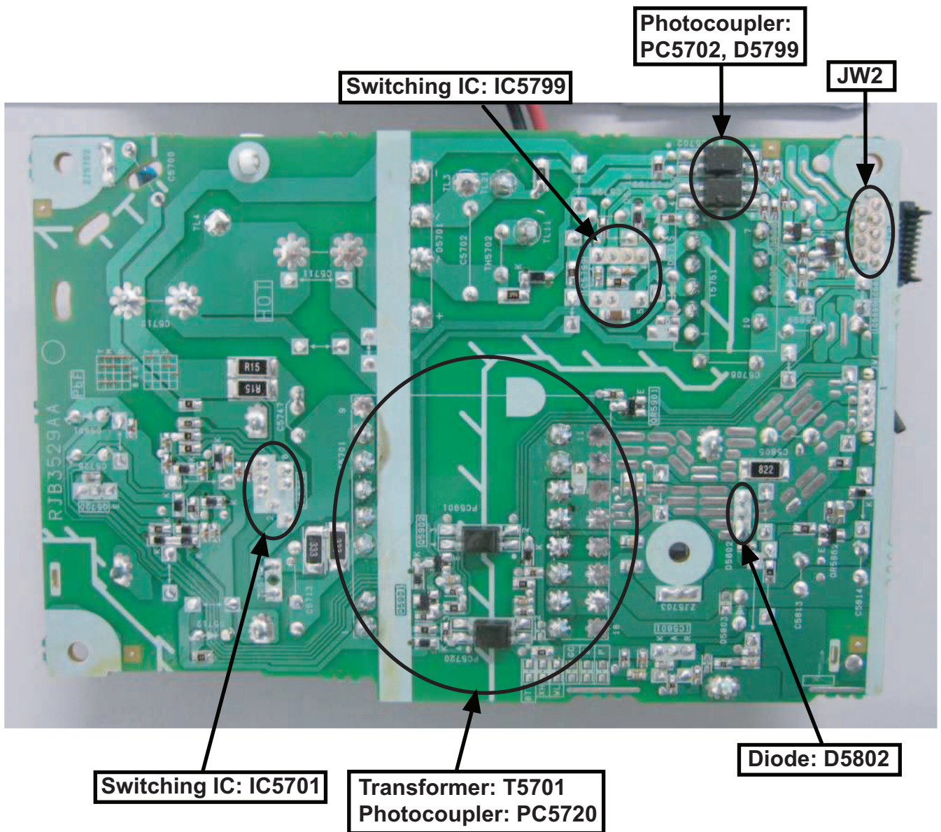
Fig 1. SMPS P.C.B.
