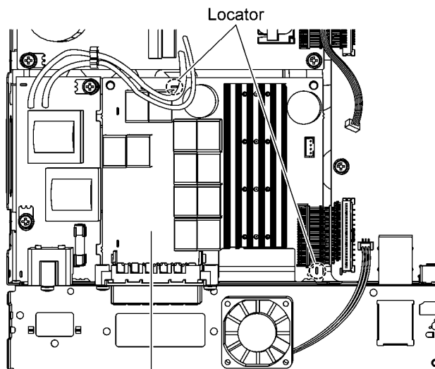
D-Amp P.C.B.
