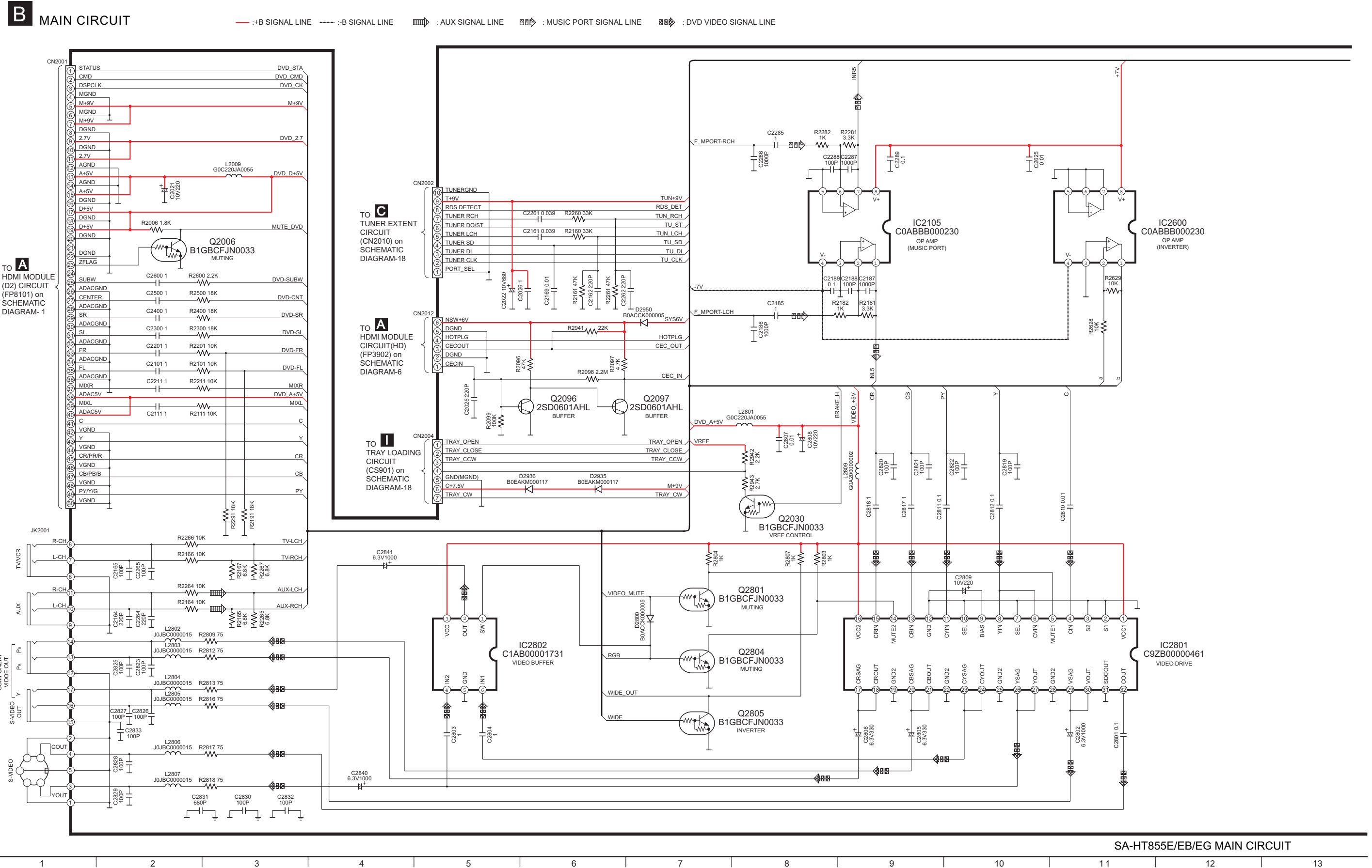
SCHEMATIC DIAGRAM-7
