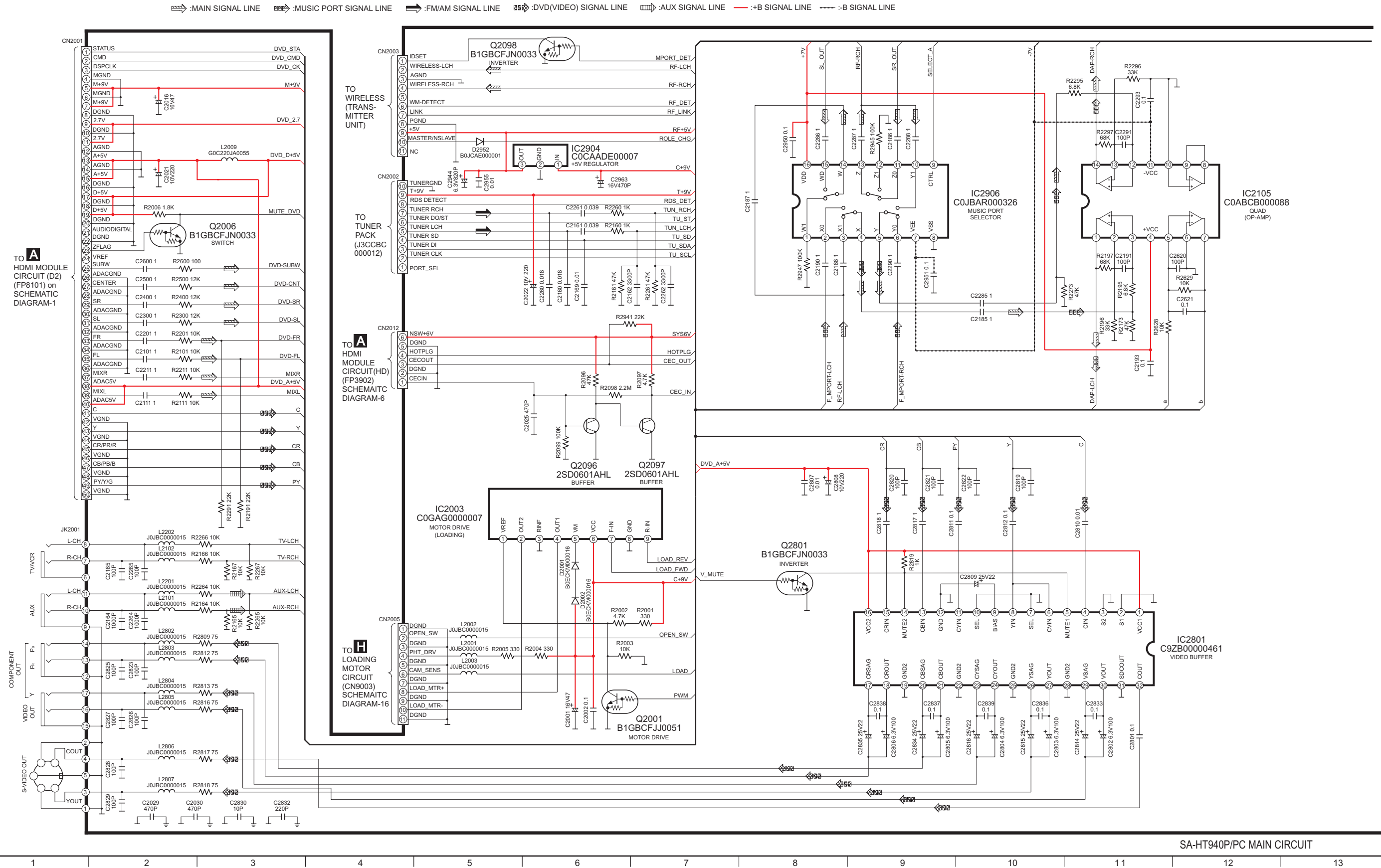
SCHEMATIC DIAGRAM-7
