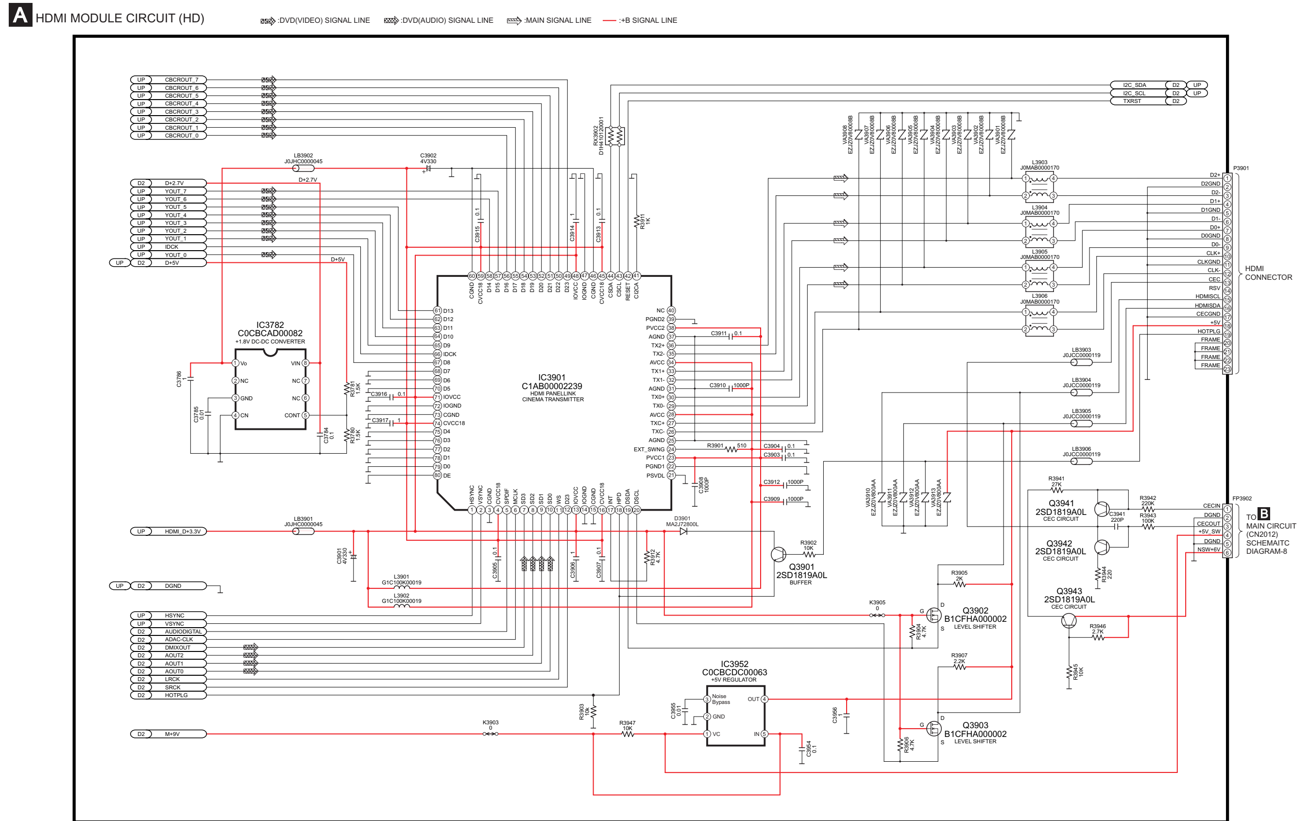
SA-HT995EE HDMI MODULE CIRCUIT (HD)
