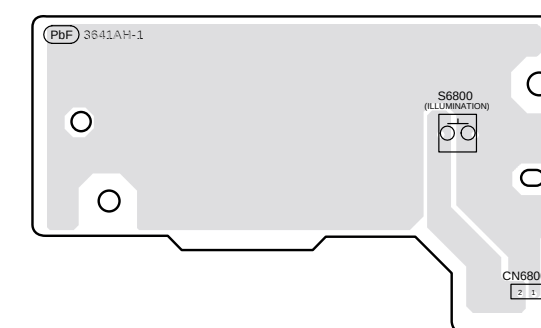
ILLUMINATION BUTTON P.C.B. (REP4883AH)
